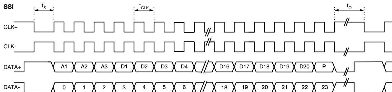
Fig. 3 - SSI Chronogram
