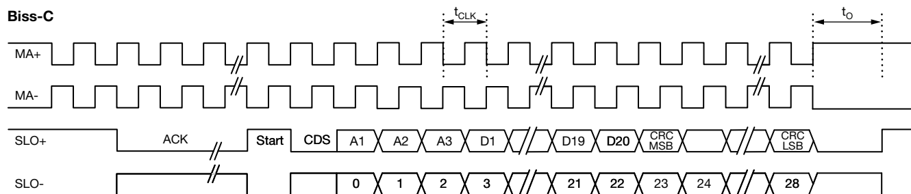
Fig. 4 - Biss-C Chronogram
