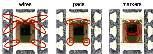
图 9-5. 封装上引脚 1 的识别特性
