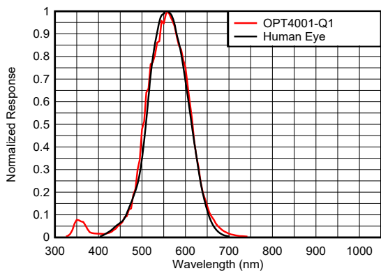
图 7-1. 光谱响应与波长间的关系
