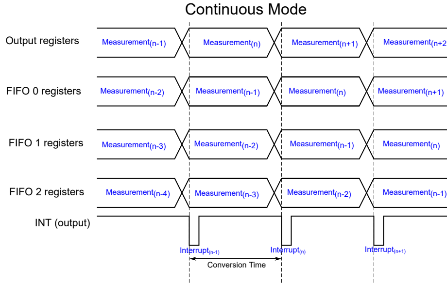
图 8-2. FIFO 寄存器数据移动
