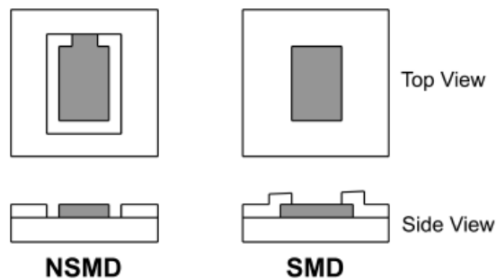
图 9-3. 阻焊层限定 (SMD) 焊盘和非阻焊层限定 (NSMD) 焊盘
