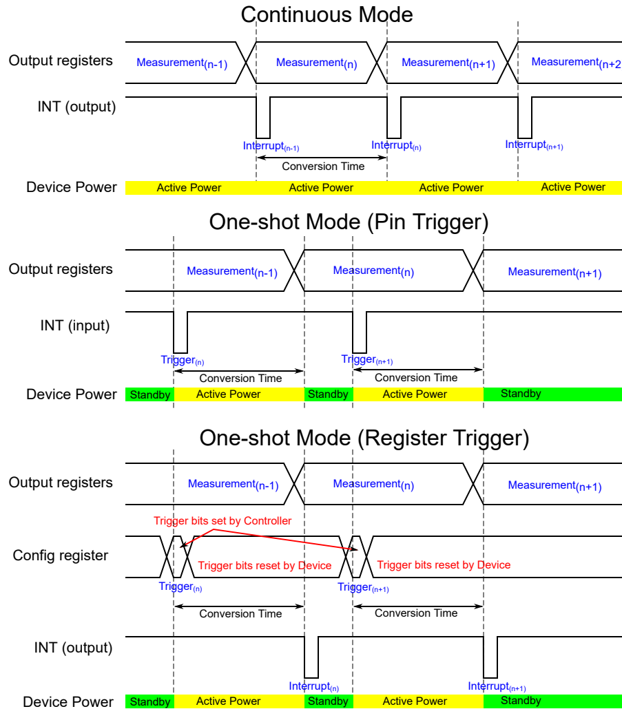
图 8-3. 不同运行模式下的时序图
