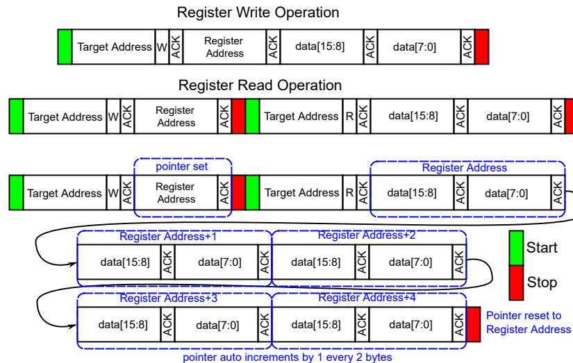
图 8-8. I 2 C 操作
