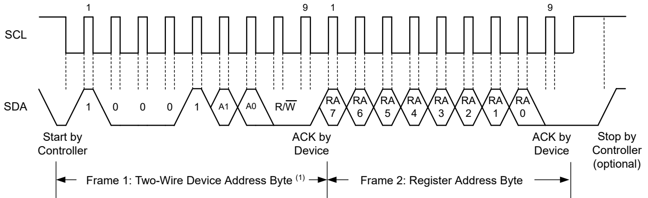
图 8-5. 设置 I 2 C 寄存器地址
