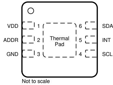
图 6-1. DNP 封装、6 引脚 USON (顶视图)
