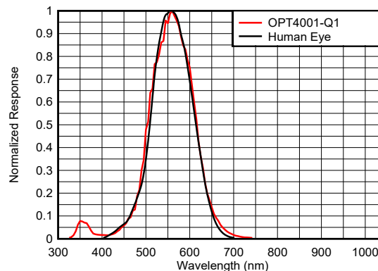
光谱响应： OPT4001-Q1 和人眼
