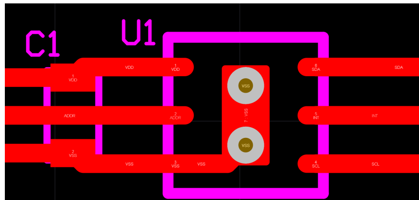
图 9-6. DNP 封装的布局示例
