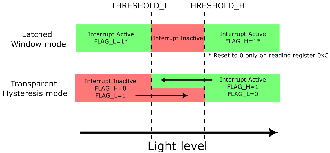
图 8-4. 中断引脚状态 (INT_CFG = 0 设置) 和寄存器标志行为
