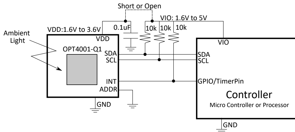
图 8-1. OPT4001-Q1 的功能方框图
