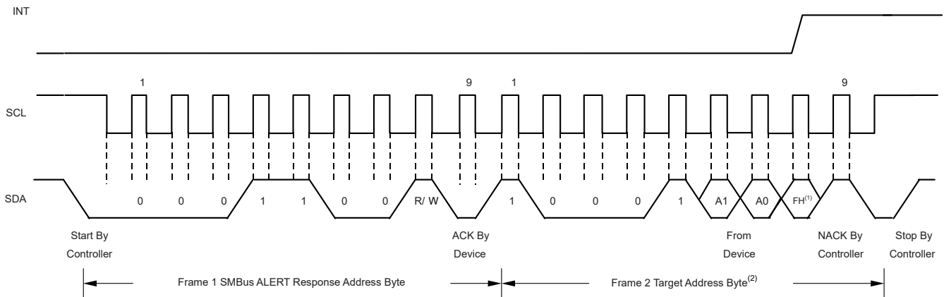
图 8-9. SMBus 警报响应时序图
