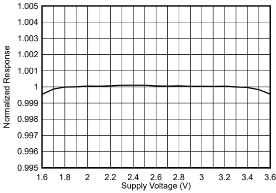
图 7-7. 器件响应与电源间的关系
