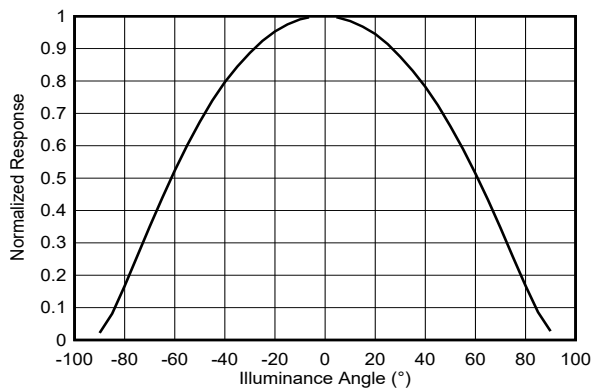
图 7-2. 器件响应与照明角度间的关系
