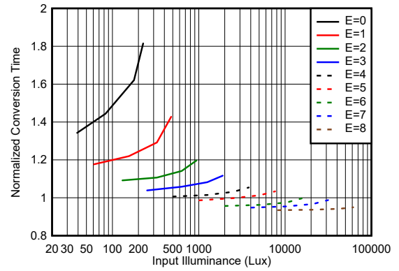
图 7-8. 600 \mu\text{s} 时的转换时间与输入照度级别间的关系
