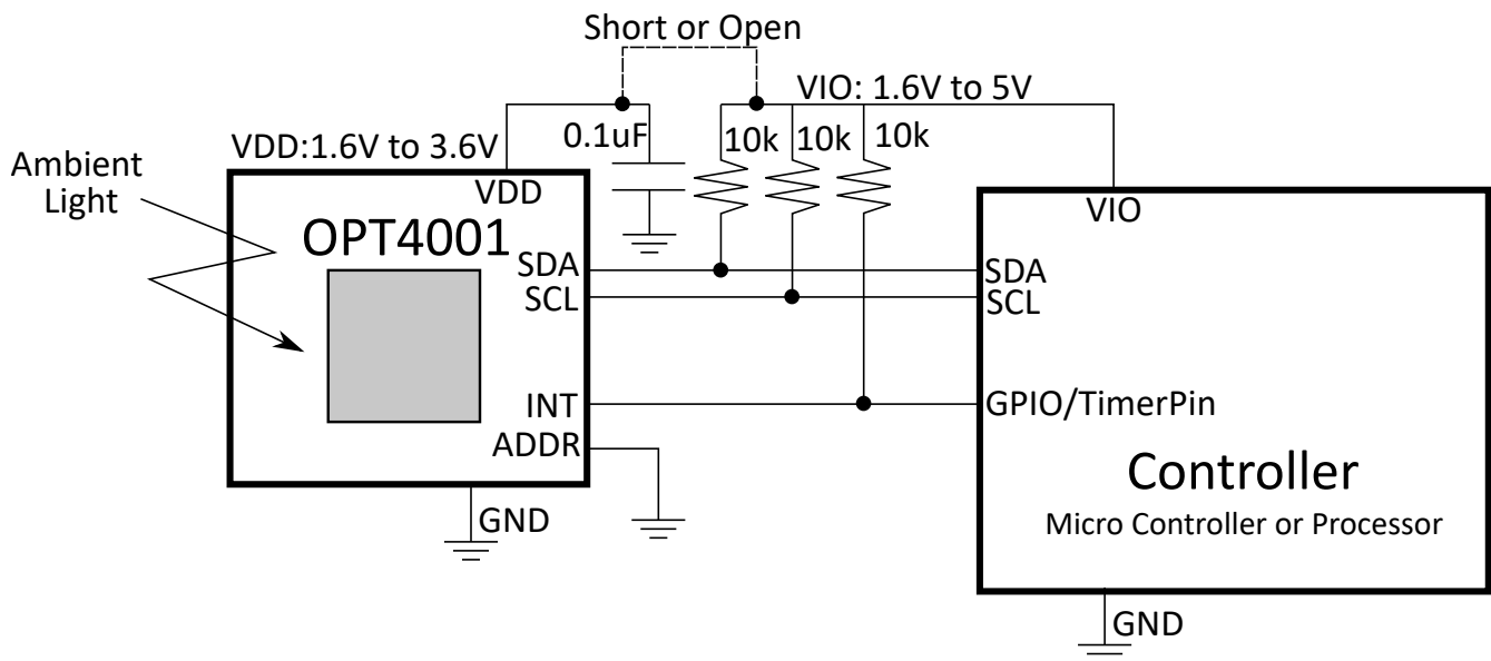
图 9-1. 典型应用原理图
