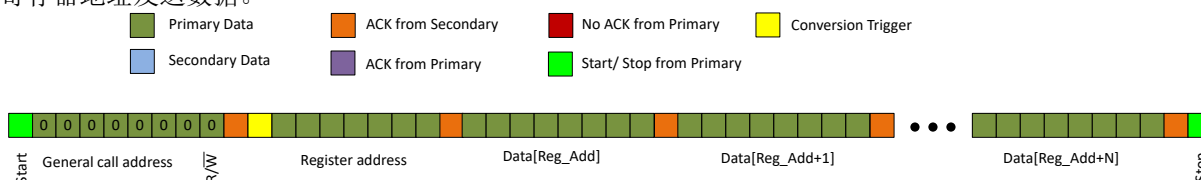
图 7-8. 通用广播 I 2 C 写入
