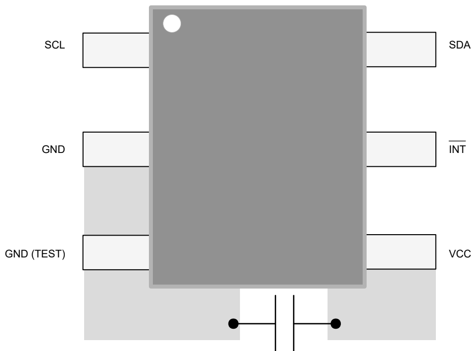
图 10-1. 布局示例 - TMAG5273
