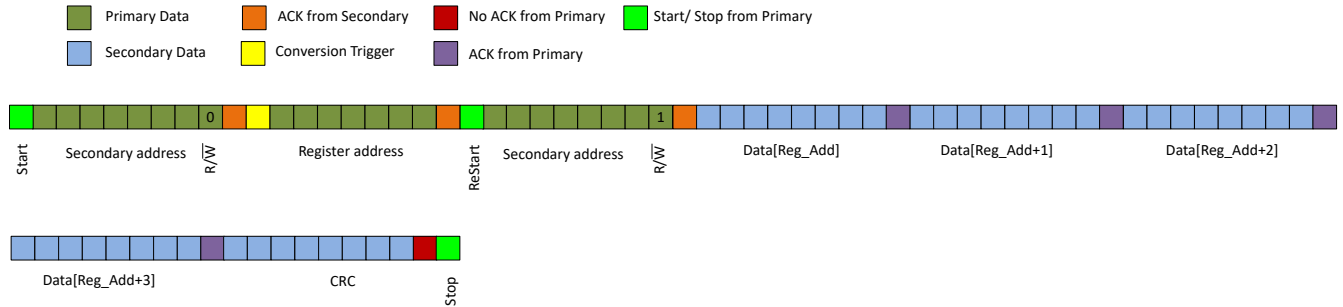
图 7-10. CRC 启用且 CRC_EN = 1b 时的标准 3 字节 I 2 C 读取
