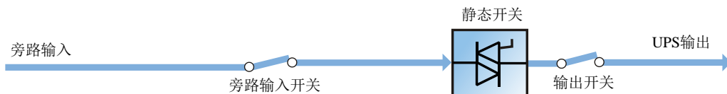
图 1-5 旁路模式运行示意图
