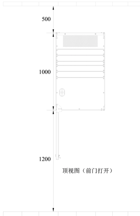
图 6-4 电池开关柜空间尺寸 (单位: mm)
