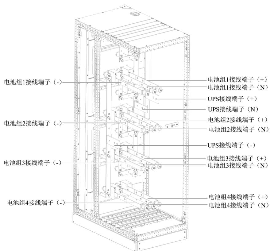
图 6-7 分 4 组电池开关柜内部接线端子说明
