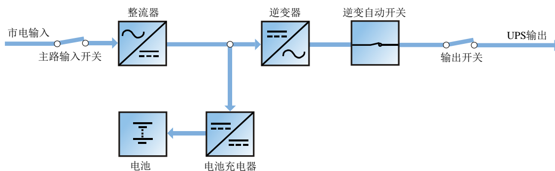
图 1-3 正常模式运行示意图
