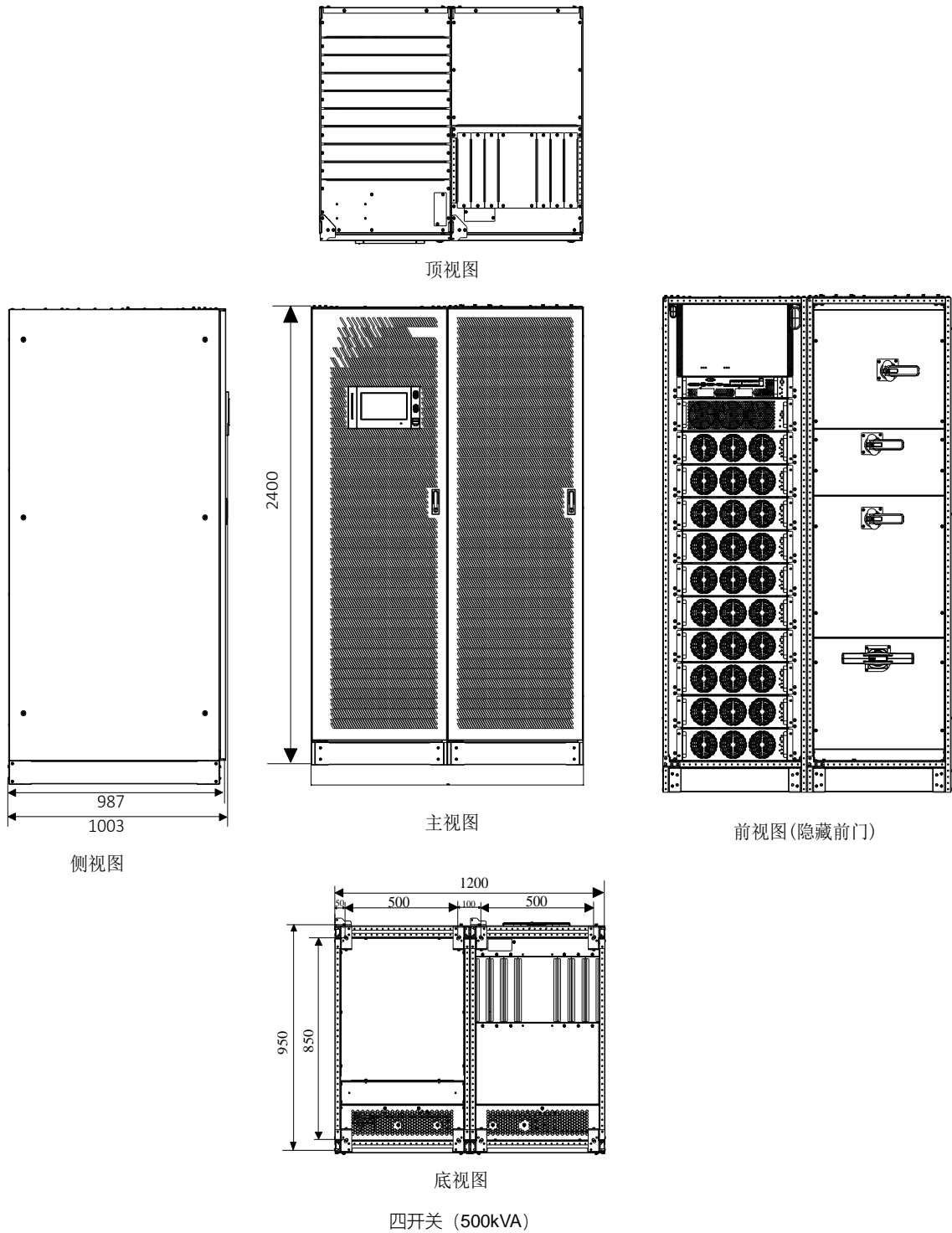
图 2-5 400~500kVA 单开关、四开关安装尺寸示意图 (单位: mm)
