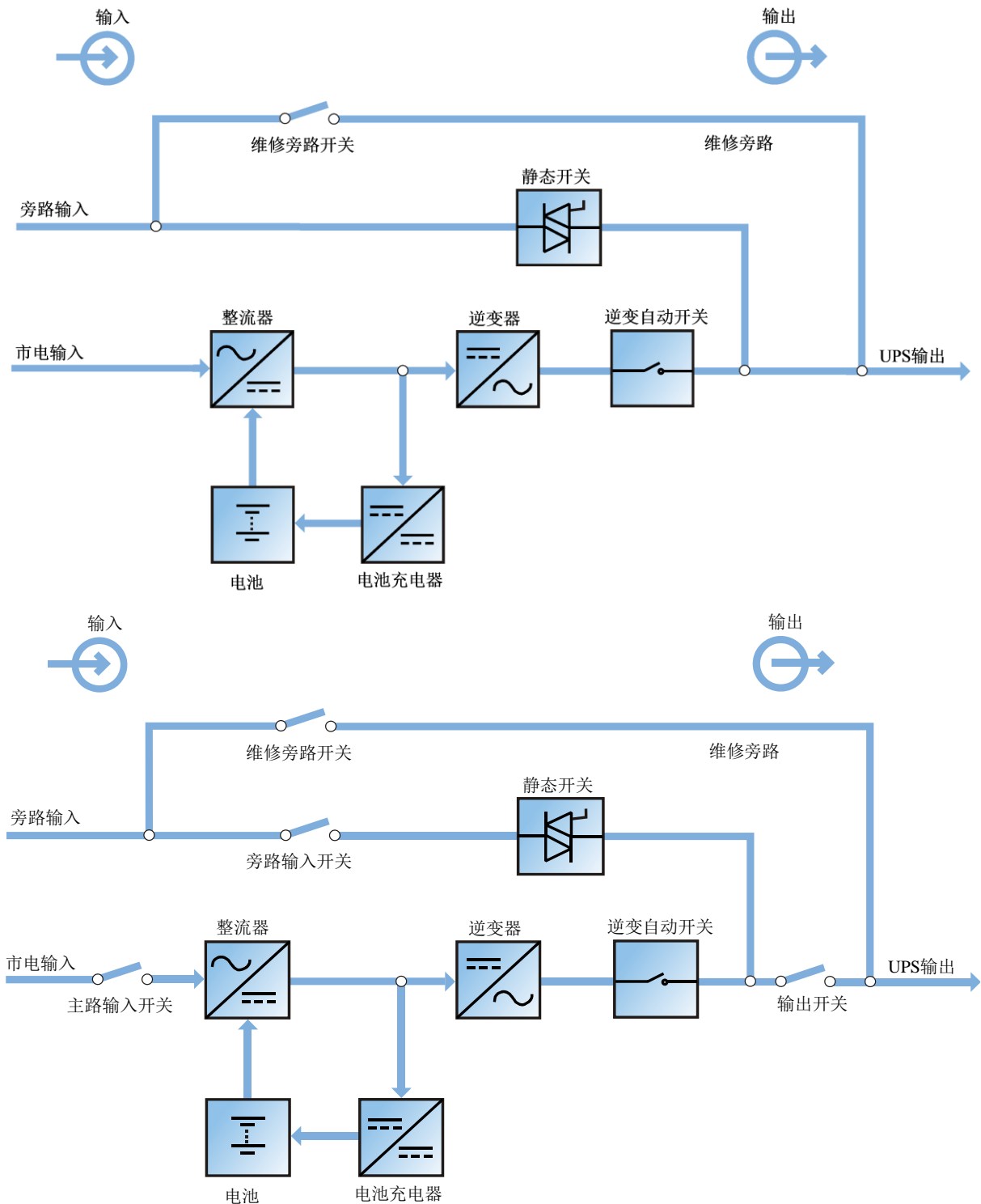
图1-1 UPS 单机工作原理框图（无开关、单开关、四开关）
