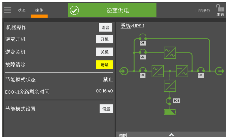
图 5-5 完成开机
