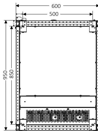
底视图
