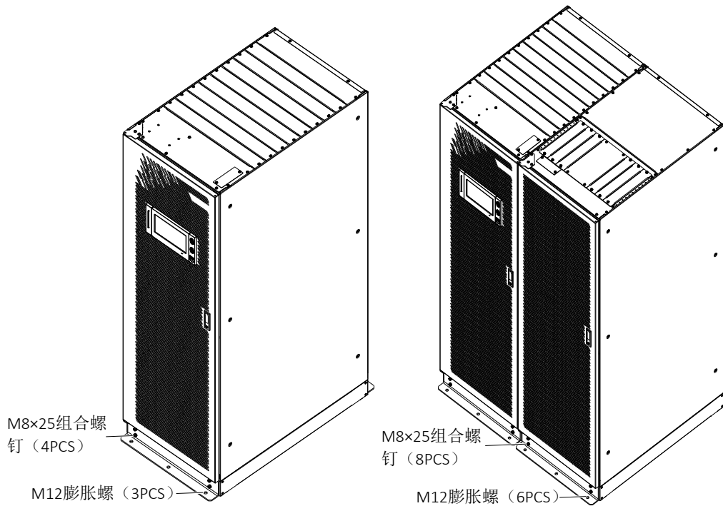
图 8-2 地震选件安装示意图（正面安装）
