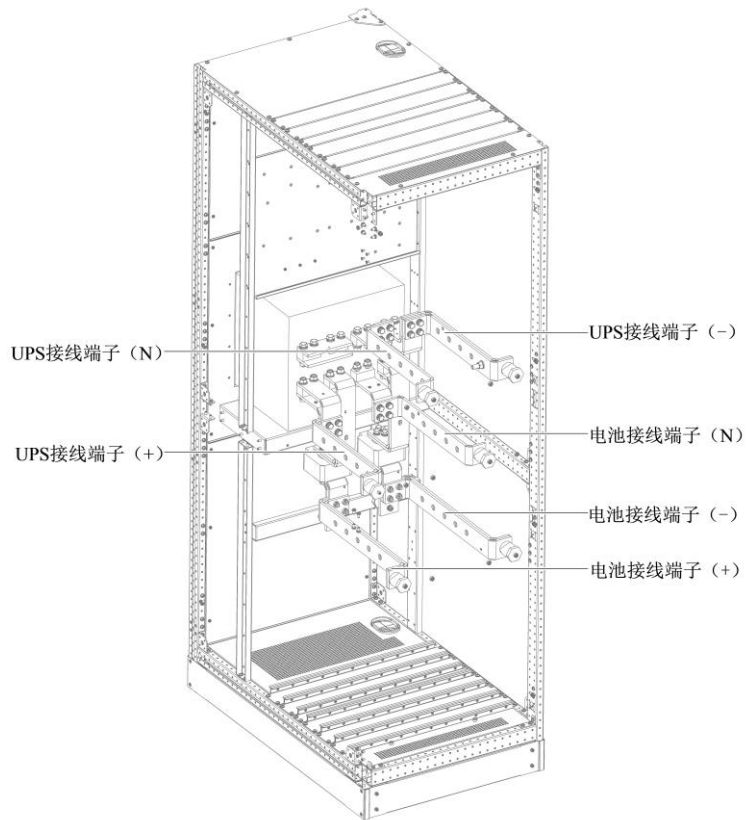
图 6-5 总体电池开关柜内部接线端子说明
