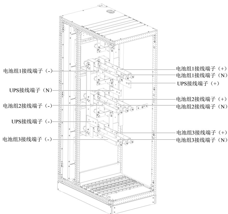
图 6-6 分 3 组电池开关柜内部接线端子说明
