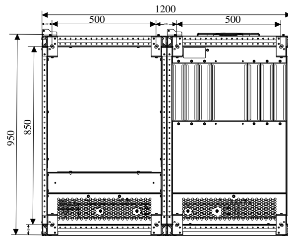
底视图
