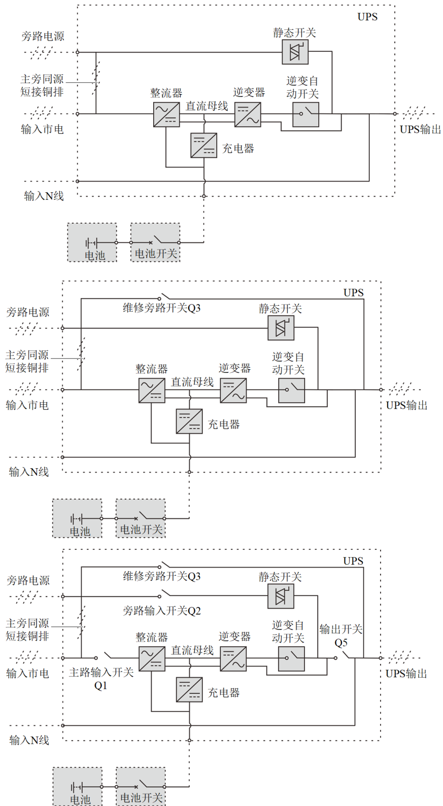
图 1-2 UPS 开关配置 (无开关、单开关、四开关)
