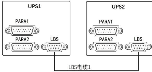
图 7-7 典型同步双母线系统的 LBS 电缆连接 (单机)
