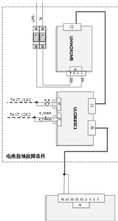
图 6-8 电池接地故障仪接线
