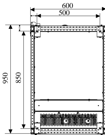
底视图
