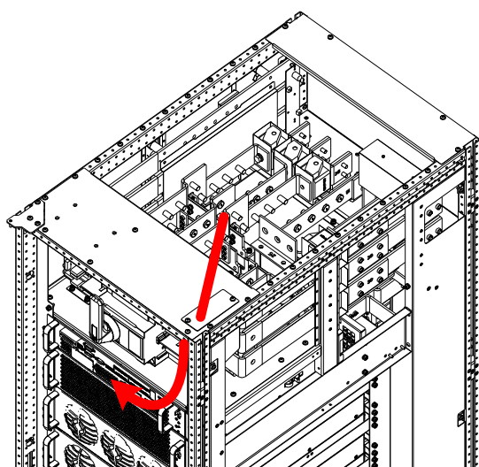
图 3-9 无开关和单开关信号电缆走线示意图
