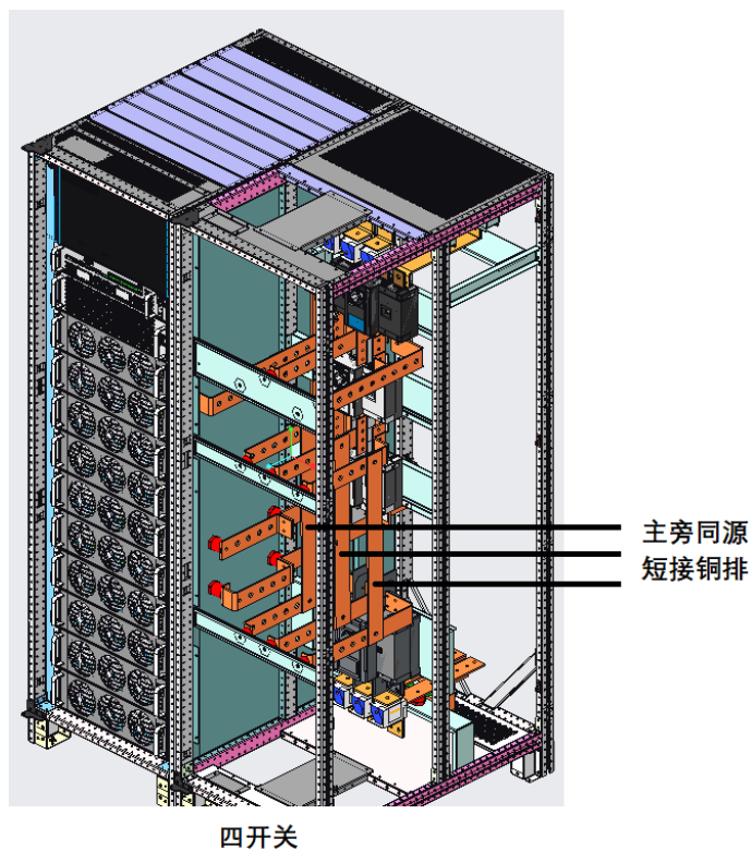
图 3-2 UPS 机柜功率电缆连接端子示意图
