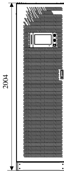
主视图
