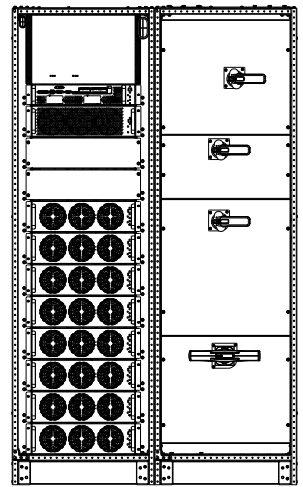
前视图(隐藏前门)
