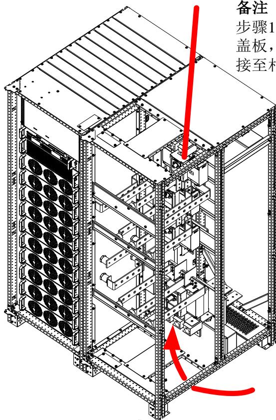
图 3-3 400~500kVA 功率电缆走线示意图
