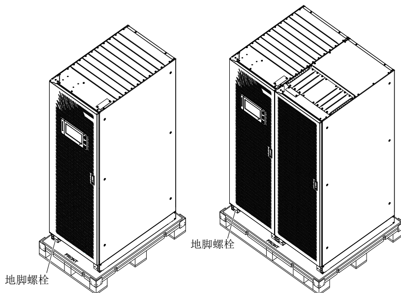
图 2-4 拆除机柜地脚螺栓
