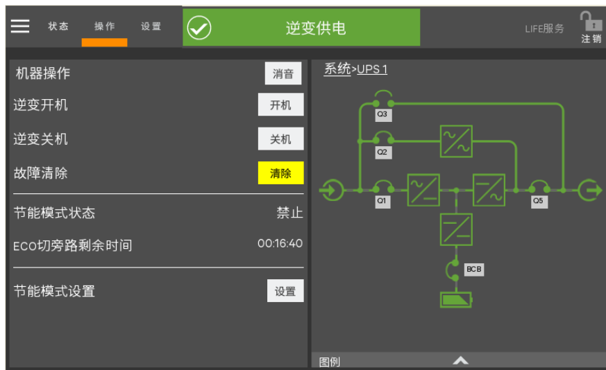
图 4-12 操作菜单
