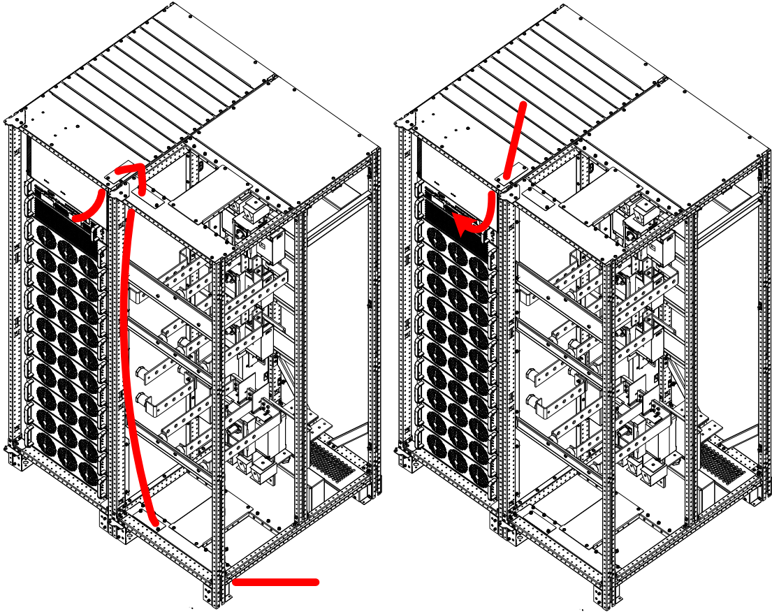
图 3-10 四开关信号电缆走线示意图 (上进线、下进线)
