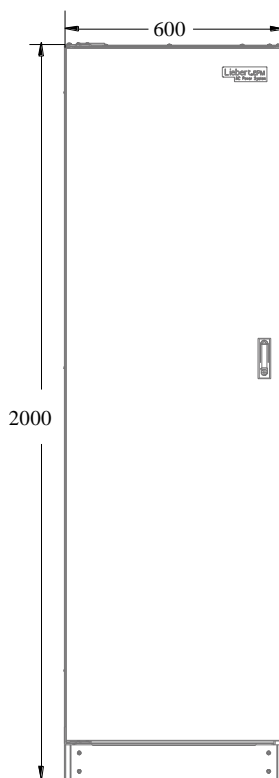
图 6-3 电池开关柜正面尺寸（单位：mm）
