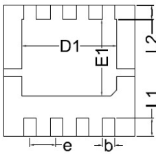
Bottom View 背面视图
