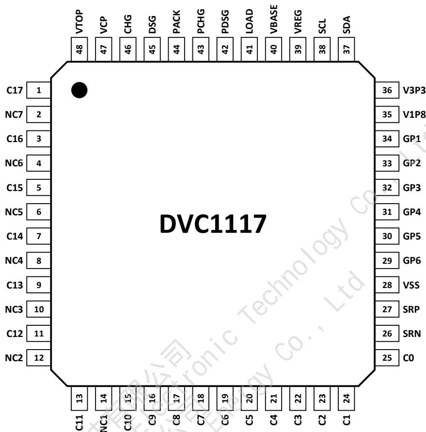
LQFP48 顶视图
