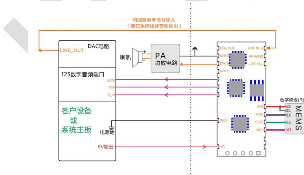
单数字麦克风连接图 (消回音模式六)
