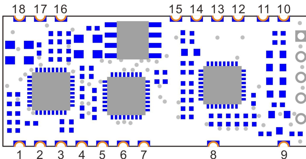
模块外形及接口示意图
