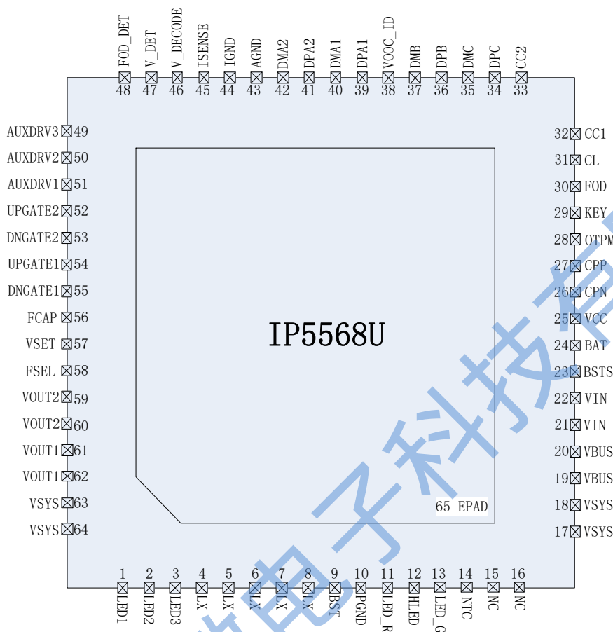
图 2 IP5568U 引脚
