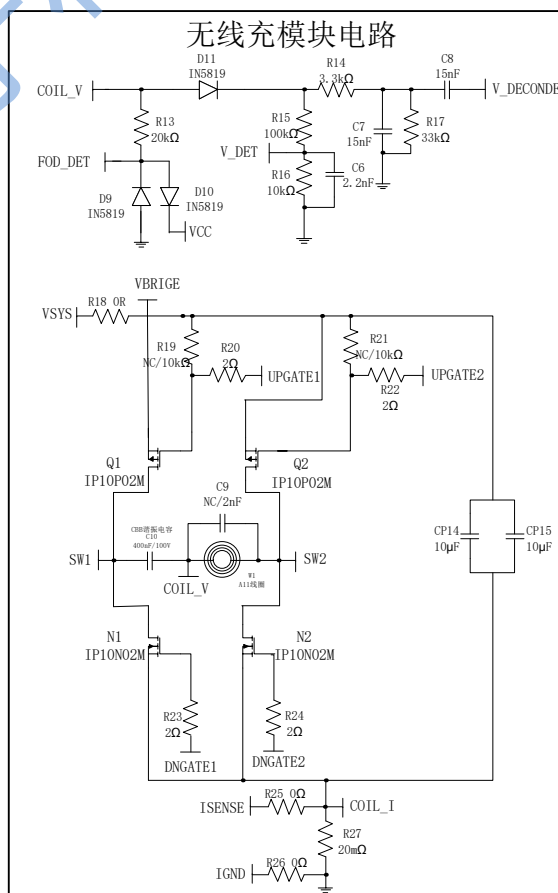
图 23 IP5568U_LED 系列应用的典型应用原理图
