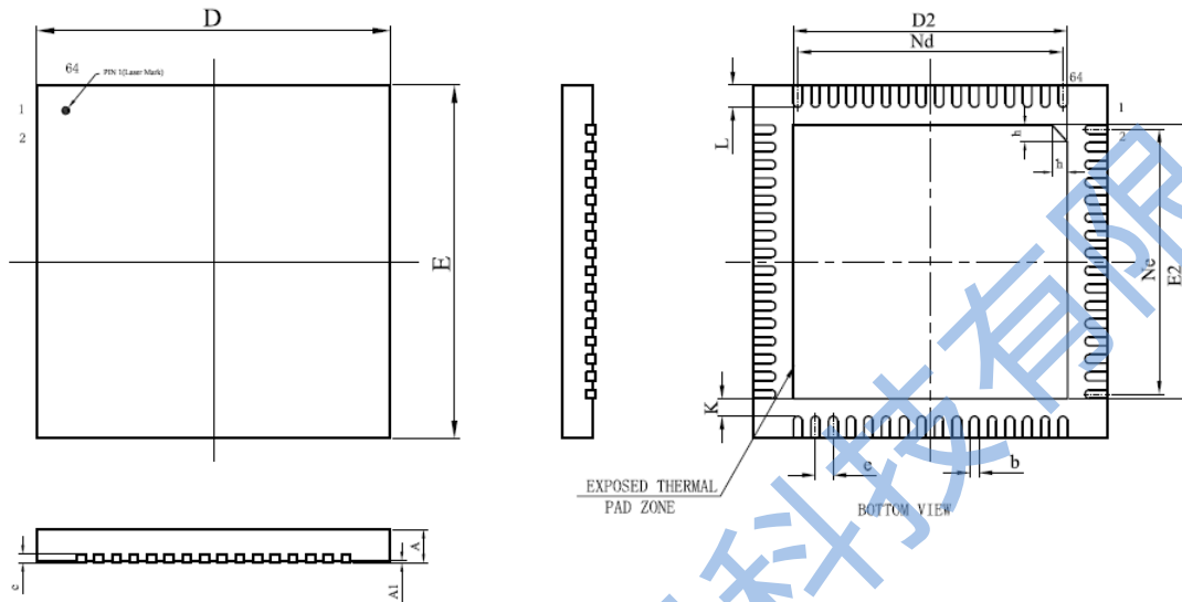
图 25 芯片封装
