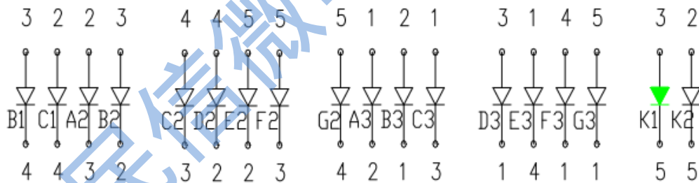
图 16 5PIN 188 数码管电路图
