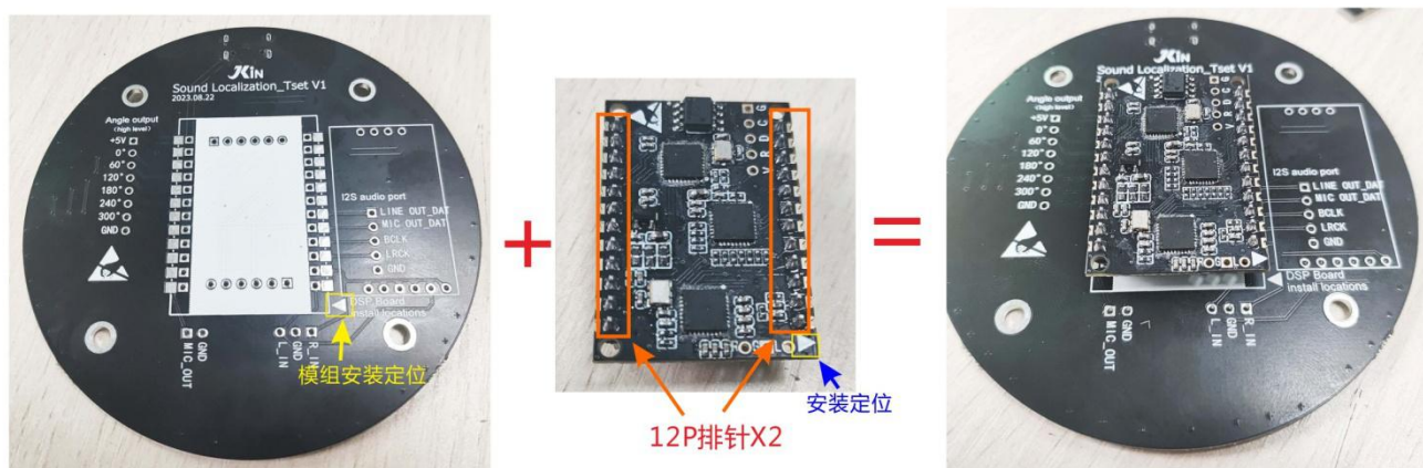
AR1105 模组与 AR-6LED 的连接实图
