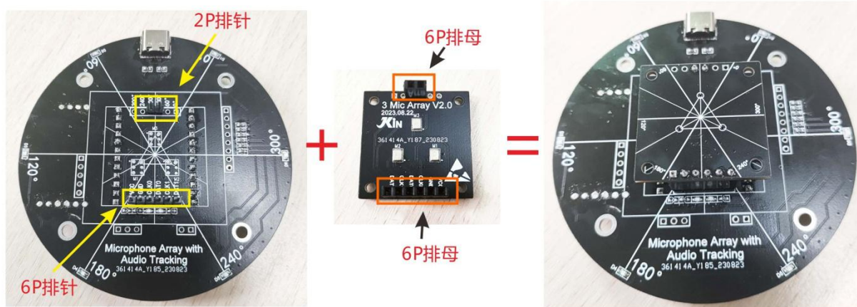
阵列麦克风板 3DMIC-291 与 AR-6LED 的连接实图
