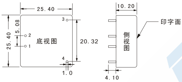
1) 外观尺寸
