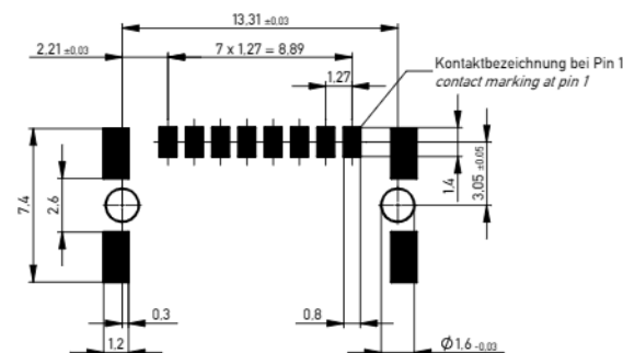
Leiterplatten-Layout für SMT PCB-Layout for SMT
