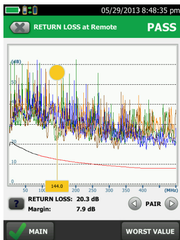
回波损耗图
