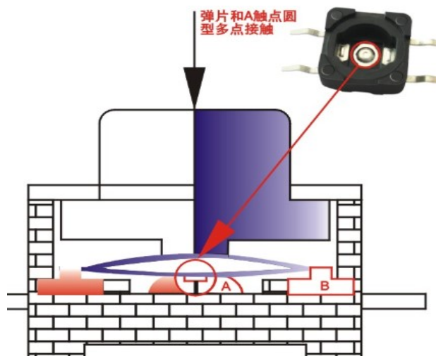
开关导通模拟图
