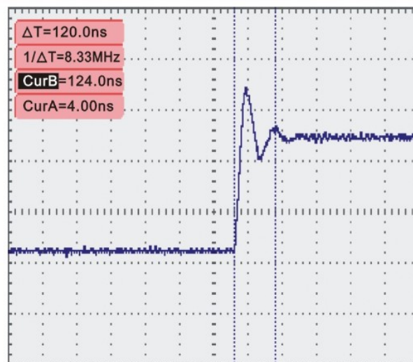
开关导通瞬间波形图
