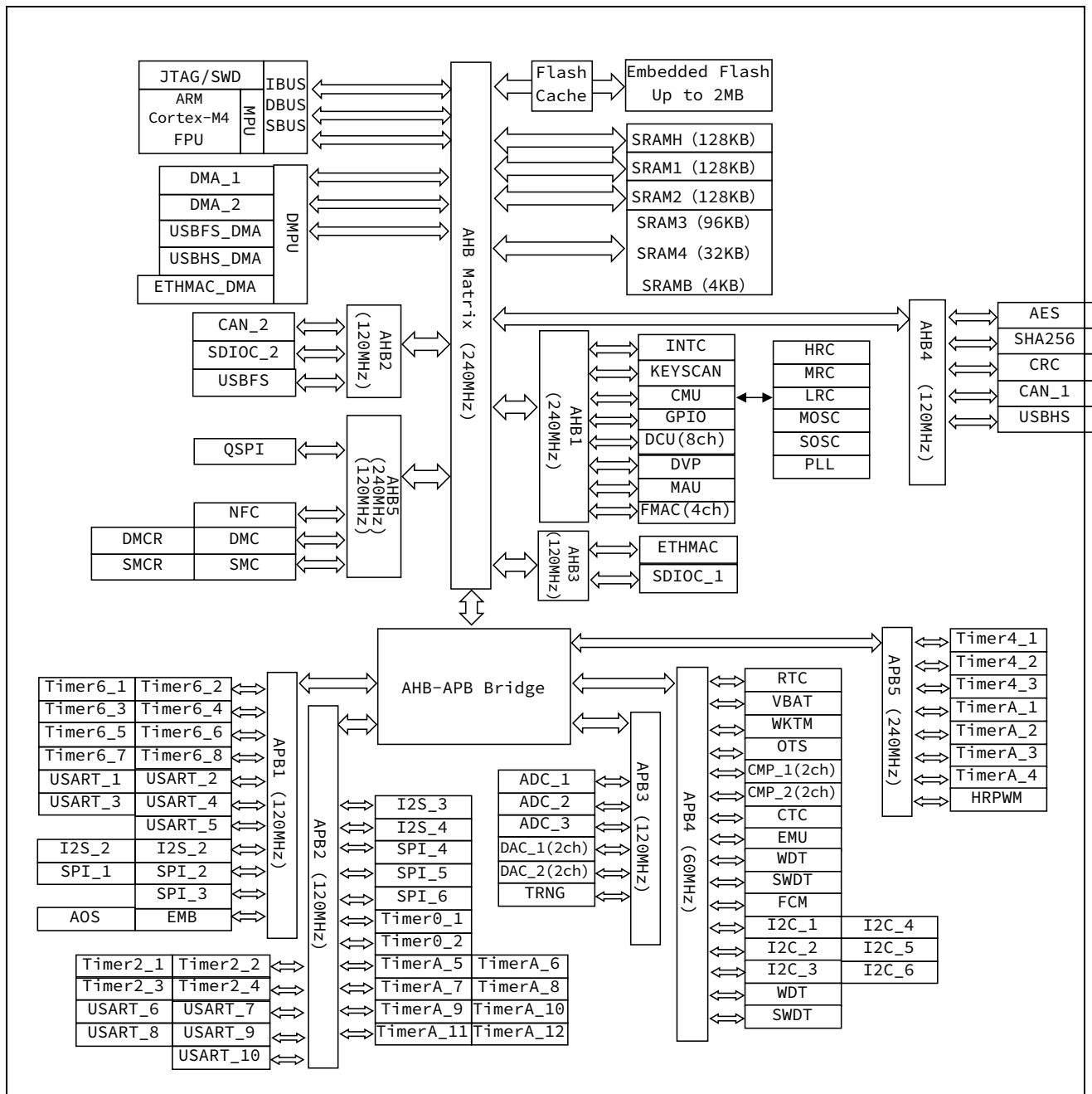
图 1-1 功能框图
