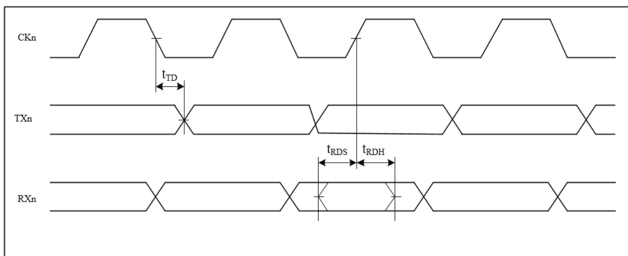
图 3-24 USART (CSI) 输入输出时序
