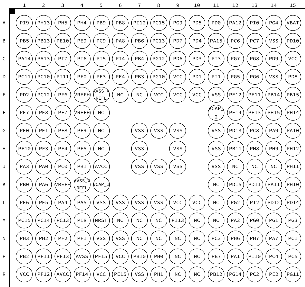
图 2-1 引脚配置图
