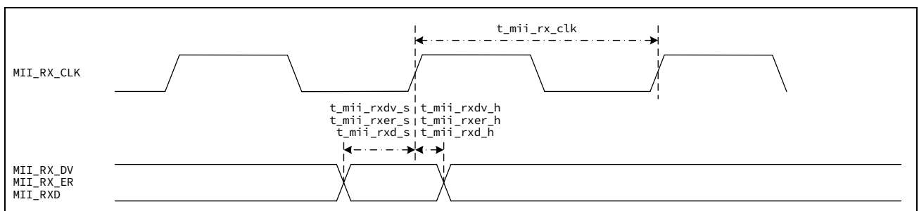
图 3-21 ETHMAC-MII 接口输入信号时序图
