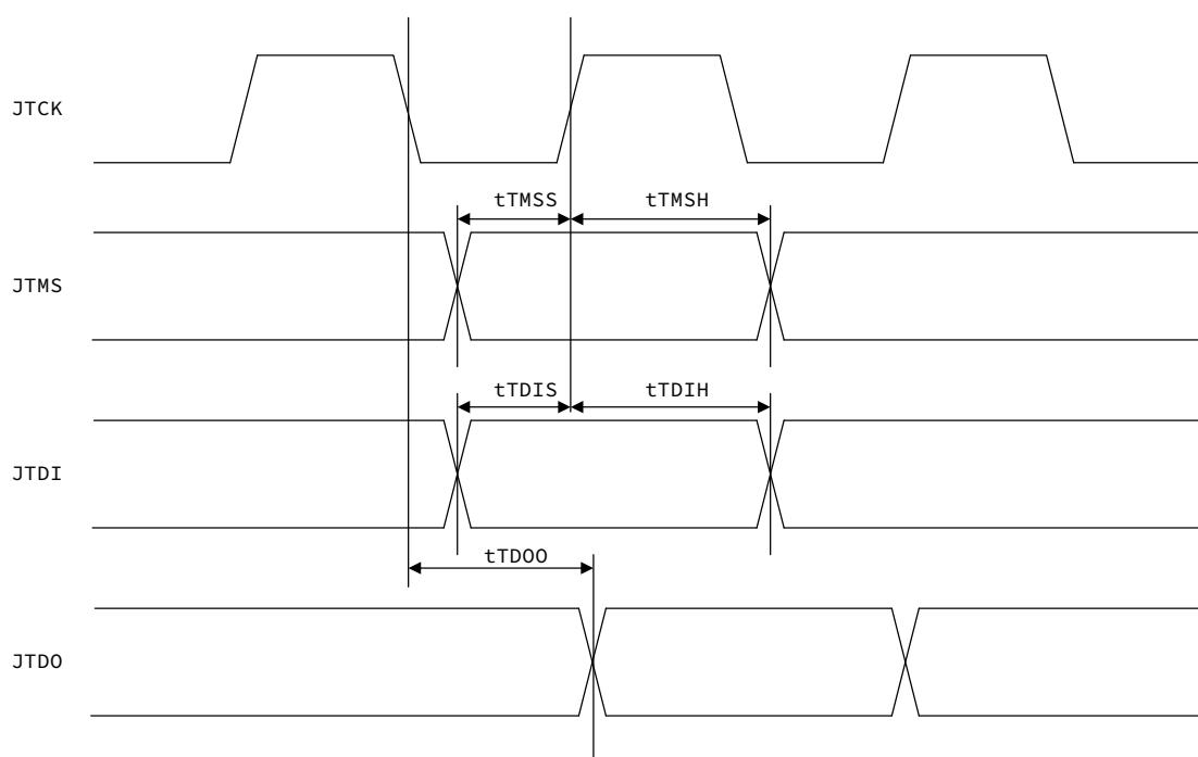
图 3-26 JTAG 输入输出
