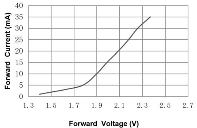
伏安特性曲线
