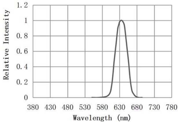
光谱分布特性曲线
