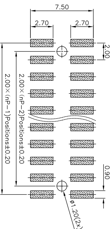
P.C.B LAYOUT
