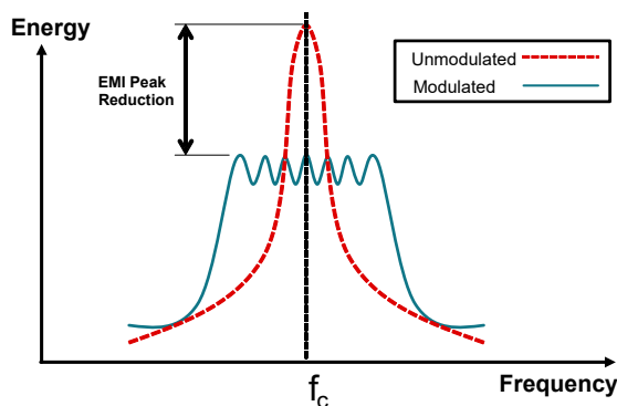
图 7-37. 展频频率调制降低 EMI
