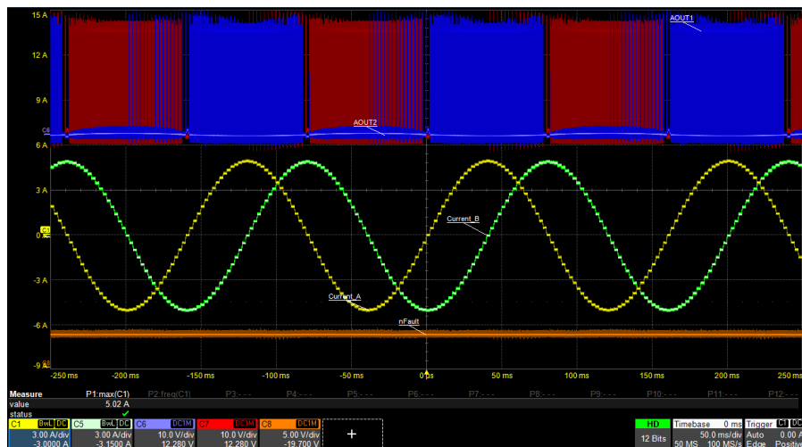
图 8-2. 在 400pps、 I_{\text{FS}} = 5\text{A} 时为 1/16 微步进
