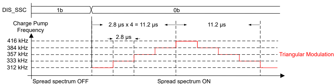
图 7-39. 电荷泵时钟的三角展频
