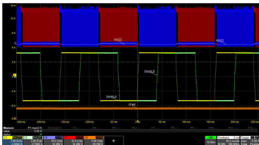
图 8-3. 25pps 下 I_{\text{FS}} = 5\text{A} 时的全步进
