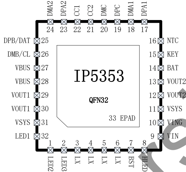
图 2 IP5353 引脚图
