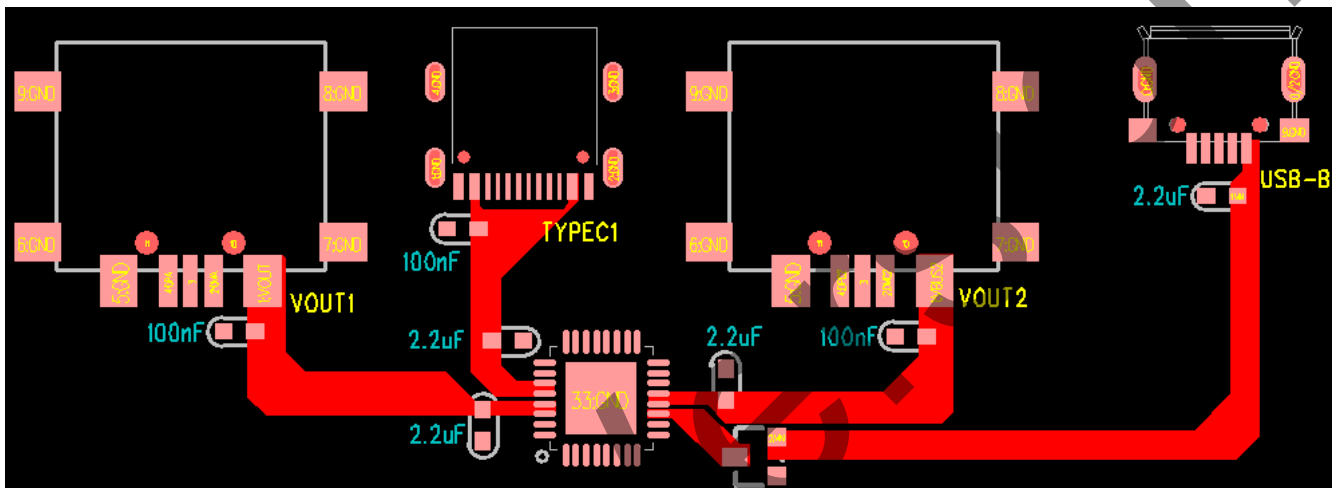
图 19 VOUT1/VOUT2/VBUS 电容位置
