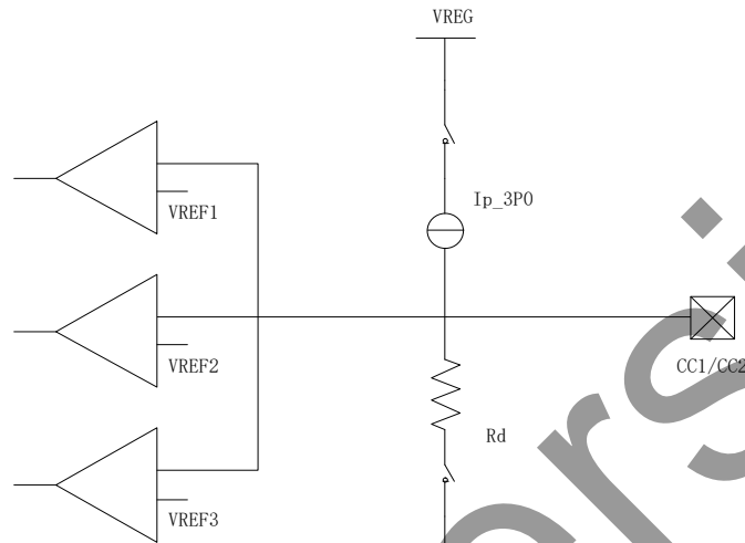
图 10 CC 内部电路
