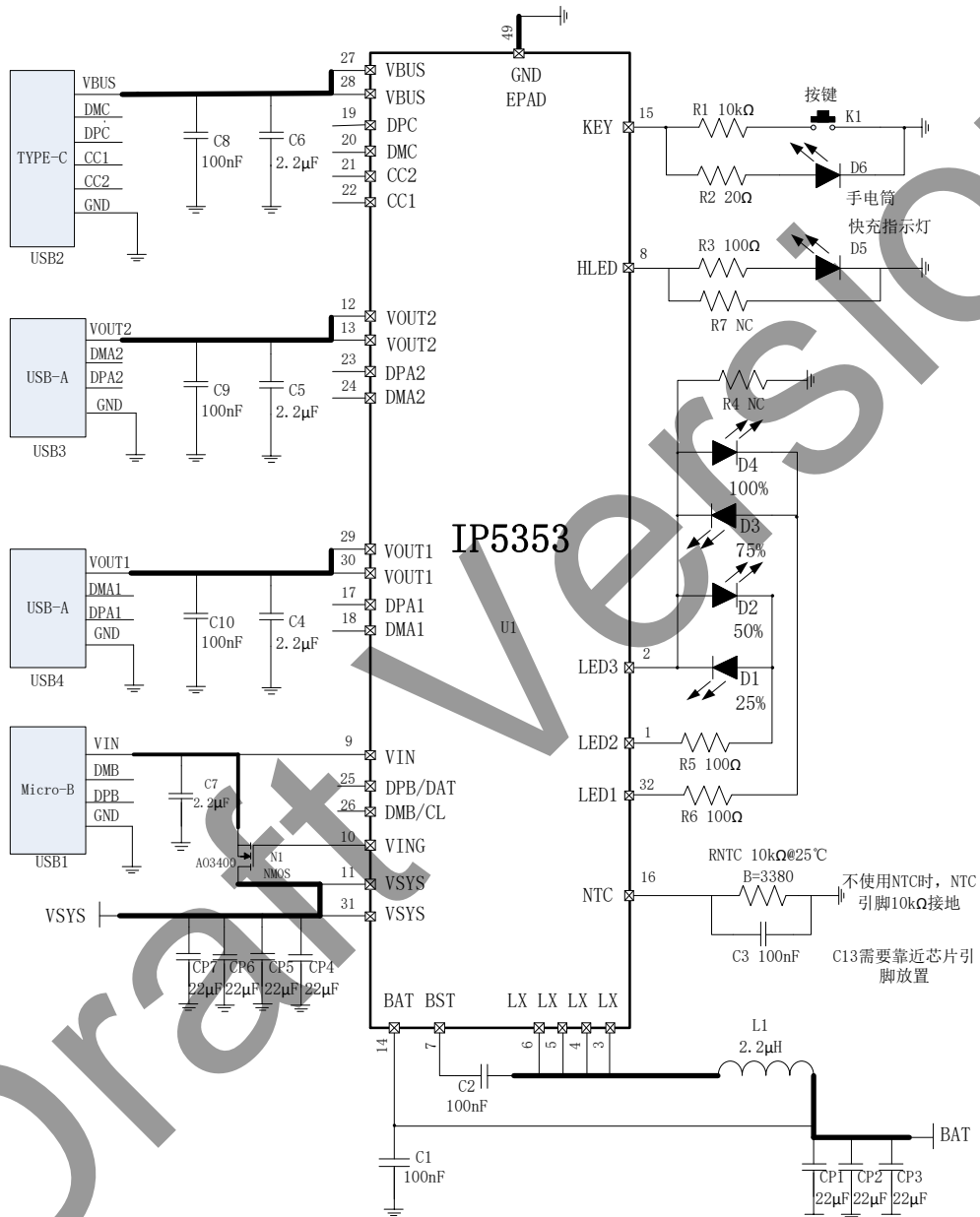
图 22 IP5353_AABC 应用原理图
