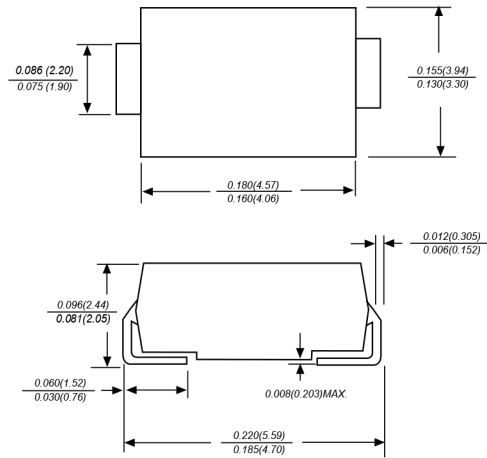
DO-214AA
