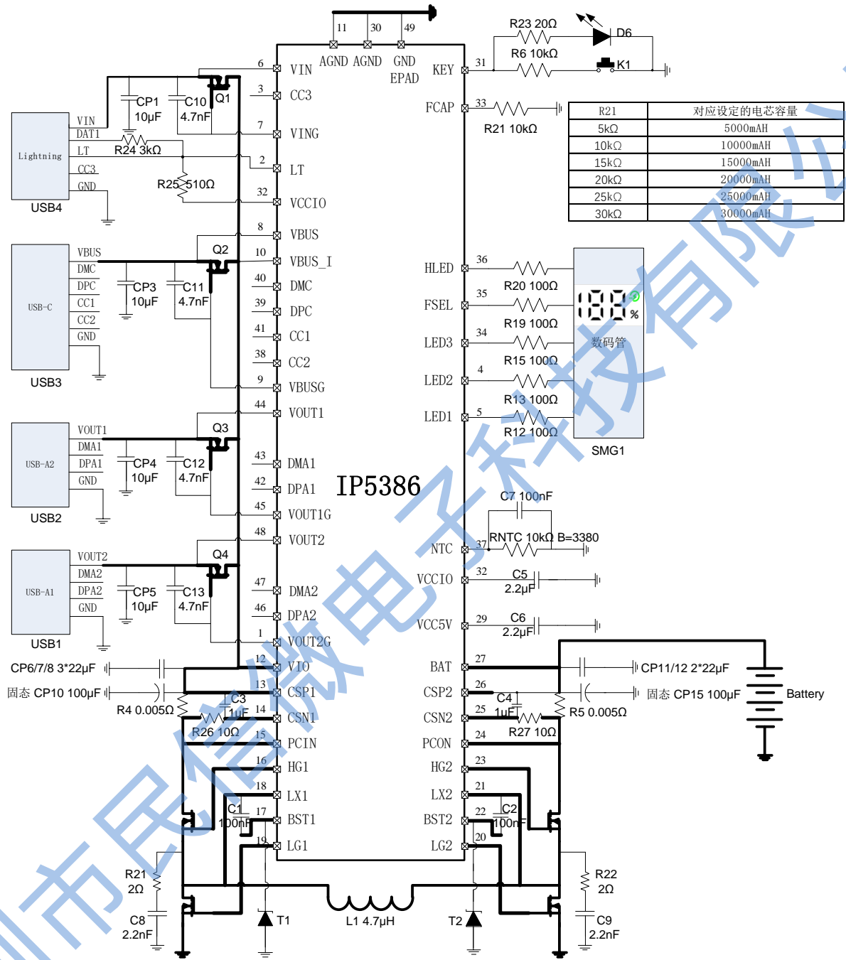
图 23 IP5386 数码管应用原理图
