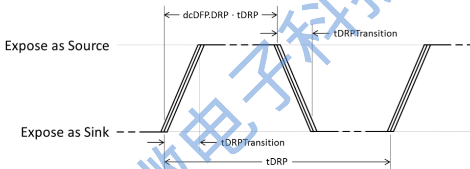
图7 USB C 检测周期
