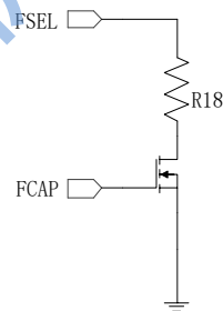
图 18 NTC 档位选择
