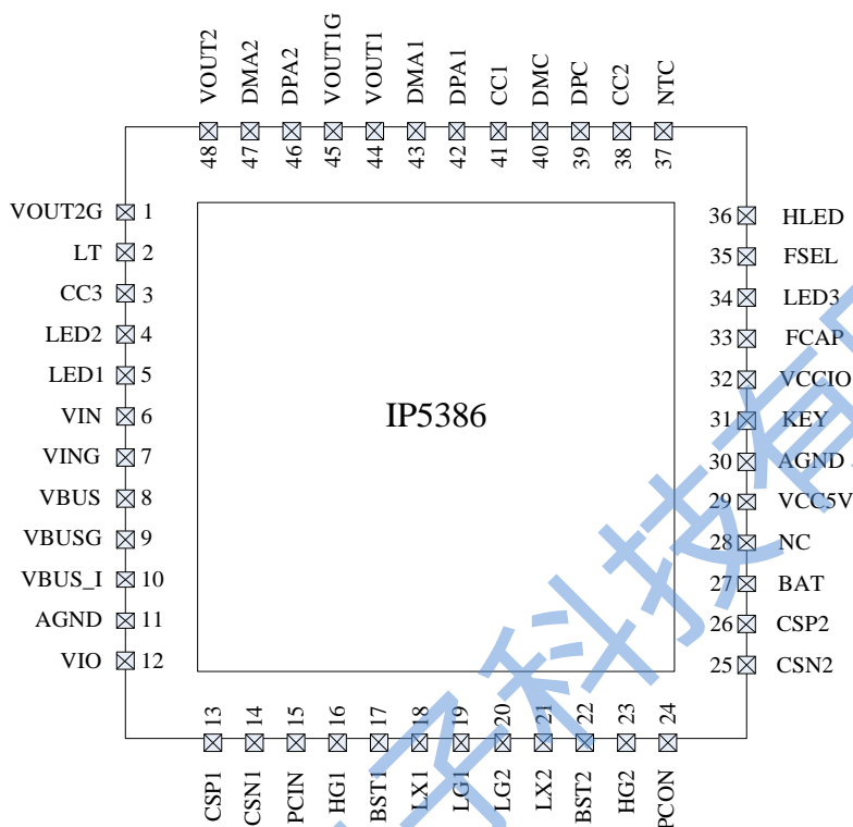
图 2 IP5386 引脚图
