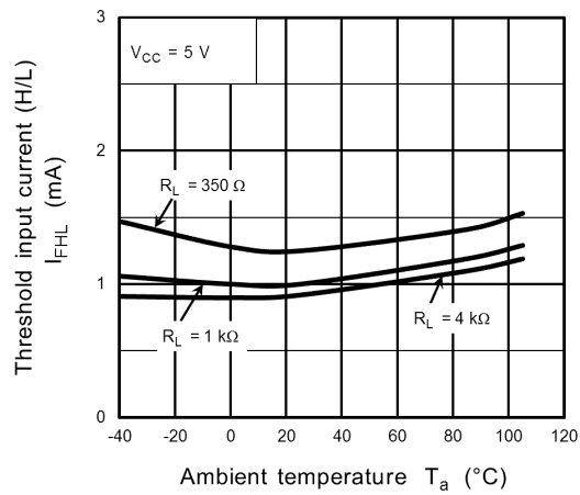
Fig. 12.2.10 I_{FHL} - T_a
