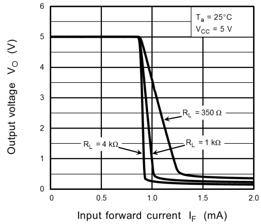
Fig. 12.2.8 V_O - I_F
