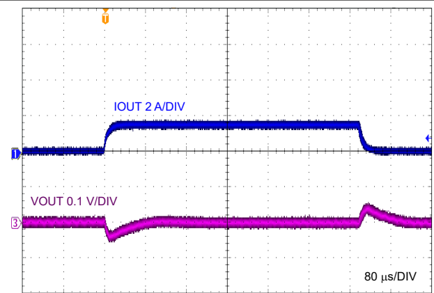
图 9-14. Load Transient, 0 A to 1.5 A
