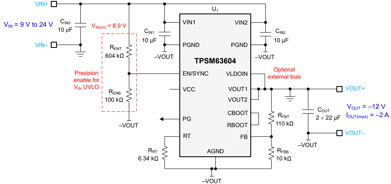
图 9-10. Circuit Schematic
