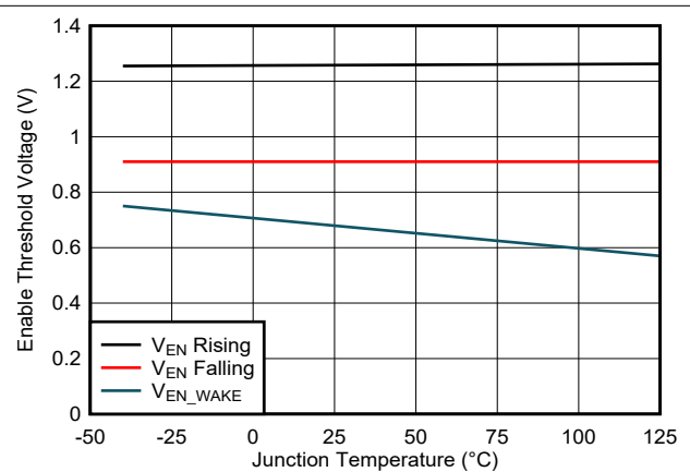
图 7-6. Enable Thresholds
