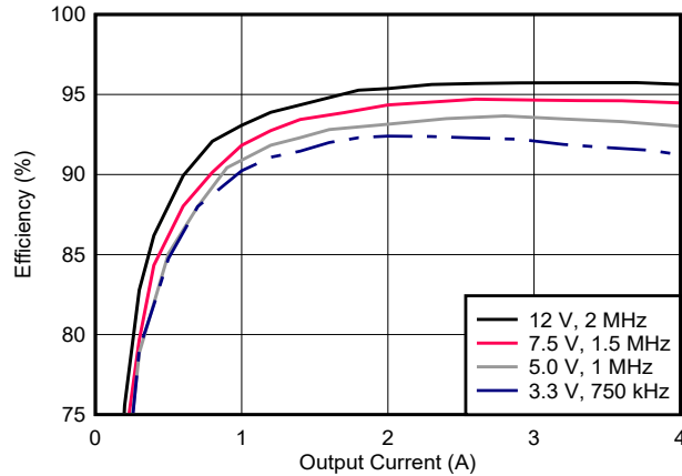
图 7-14. Efficiency
