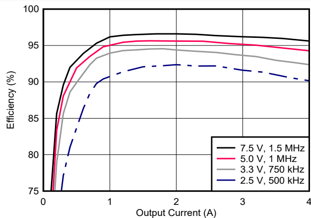
图 7-9. Efficiency
