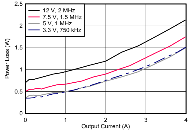
图 7-15. Power Dissipation
