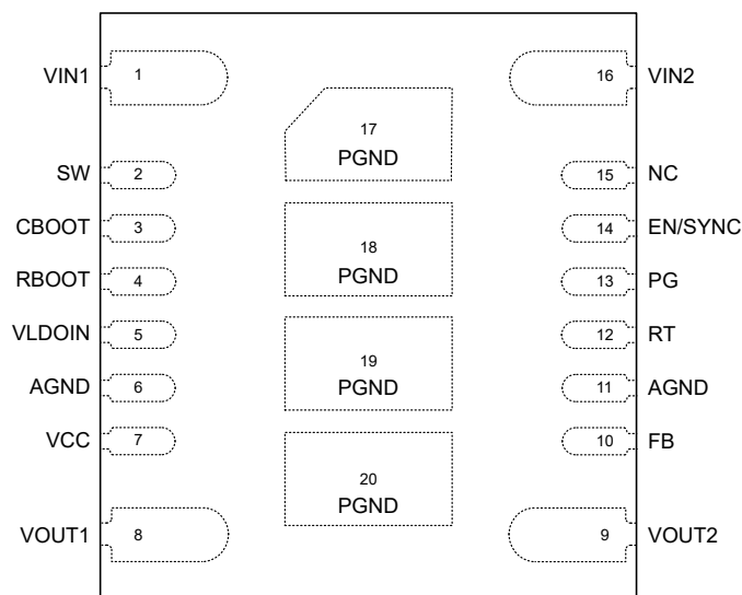
图 6-1. 20-Pin QFN RDL Package (Top View)
