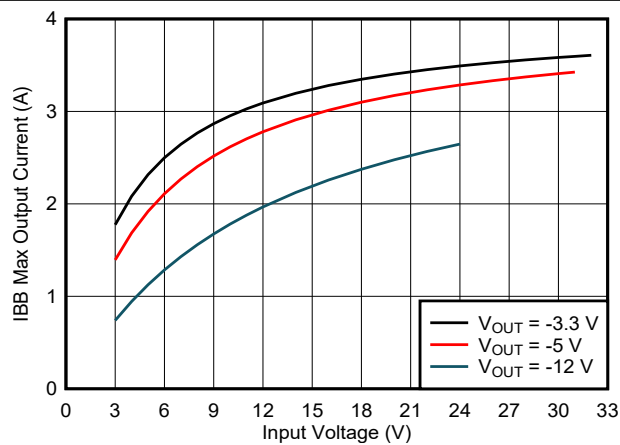
图 9-11. IBB Maximum Output Current
