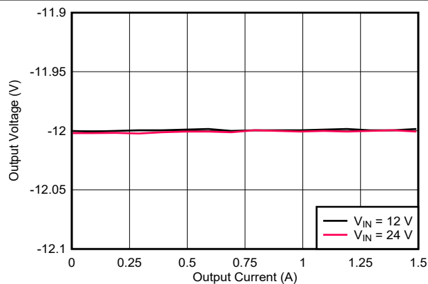
图 9-13. Load Regulation
