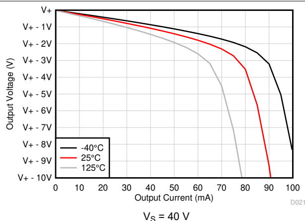
图 6-12. 输出电压摆幅与输出电流 (拉电流) 间的关系
