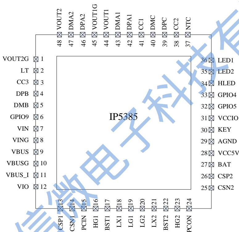
图 2 IP5385 引脚图
