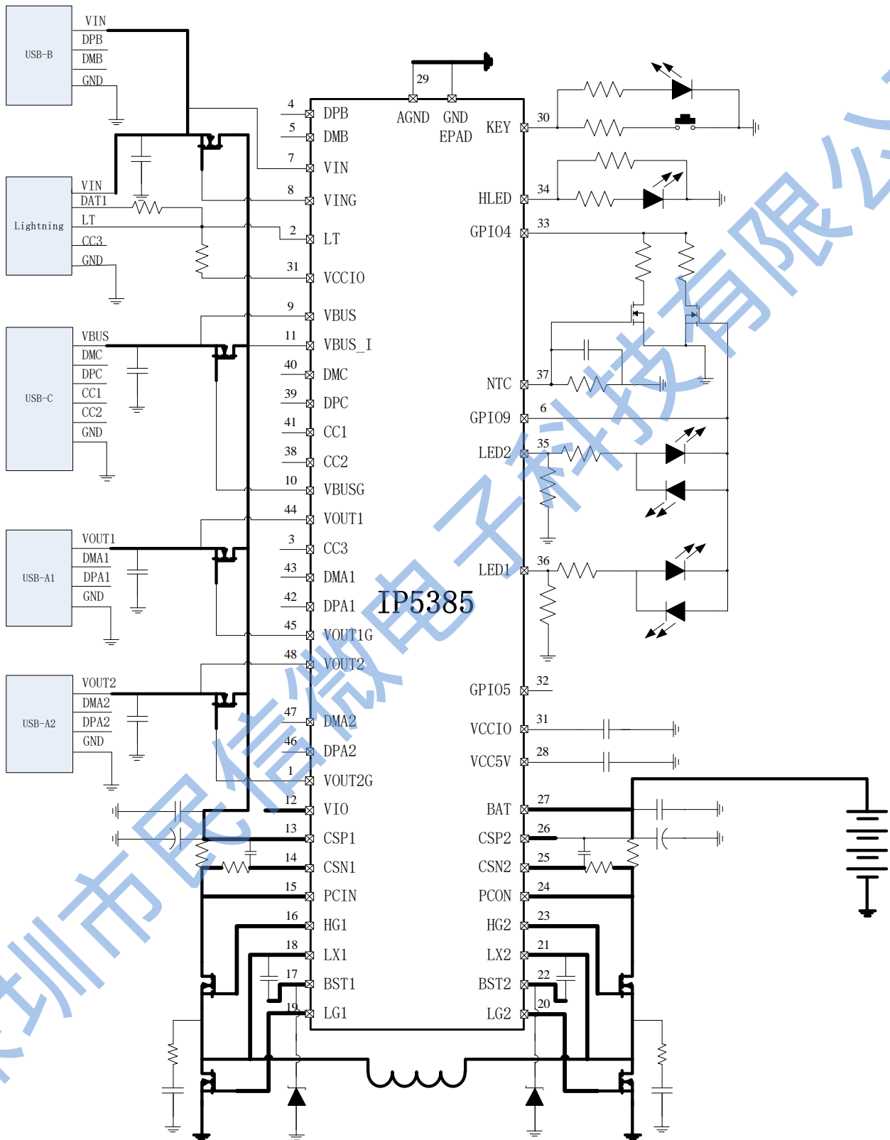
图 1 IP5385 简化应用原理图
