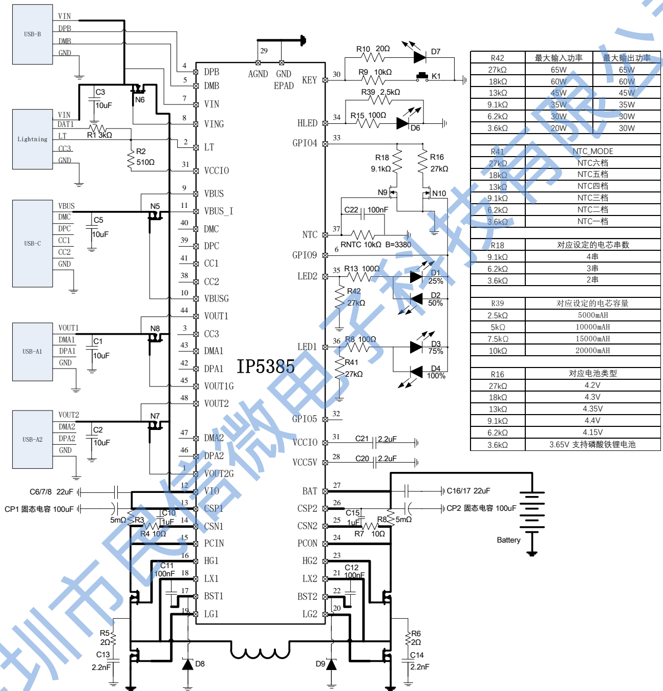
图 22 IP5385 LED 应用原理图
