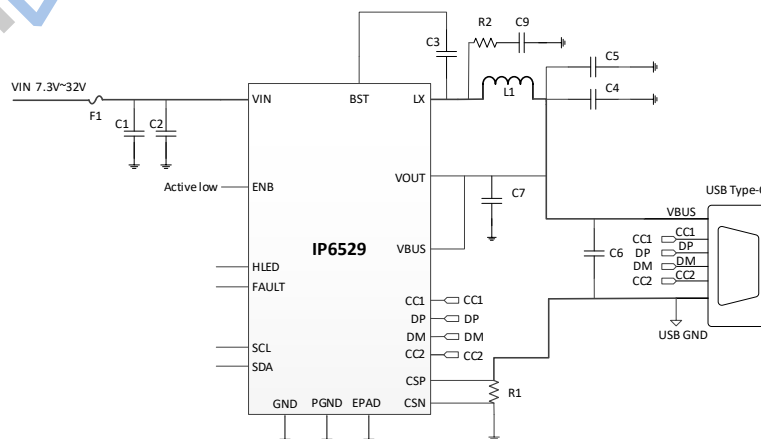
图 1 IP6529 输出简化应用原理图
