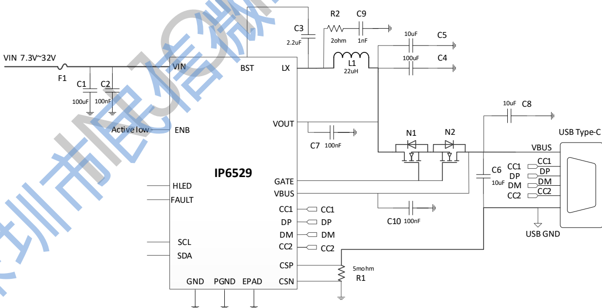
图 9 IP6529 支持外部采样电阻和路径 MOS 的 PD 快充输出应用原理图
