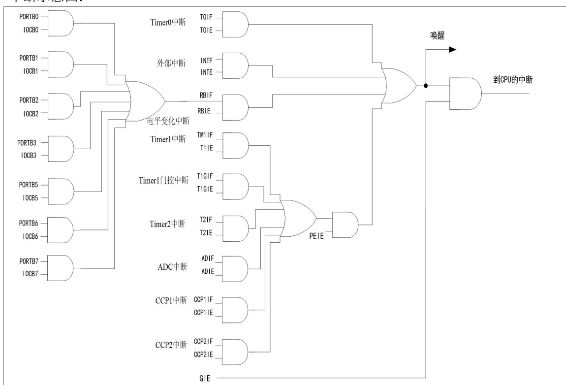
中断示意图:
