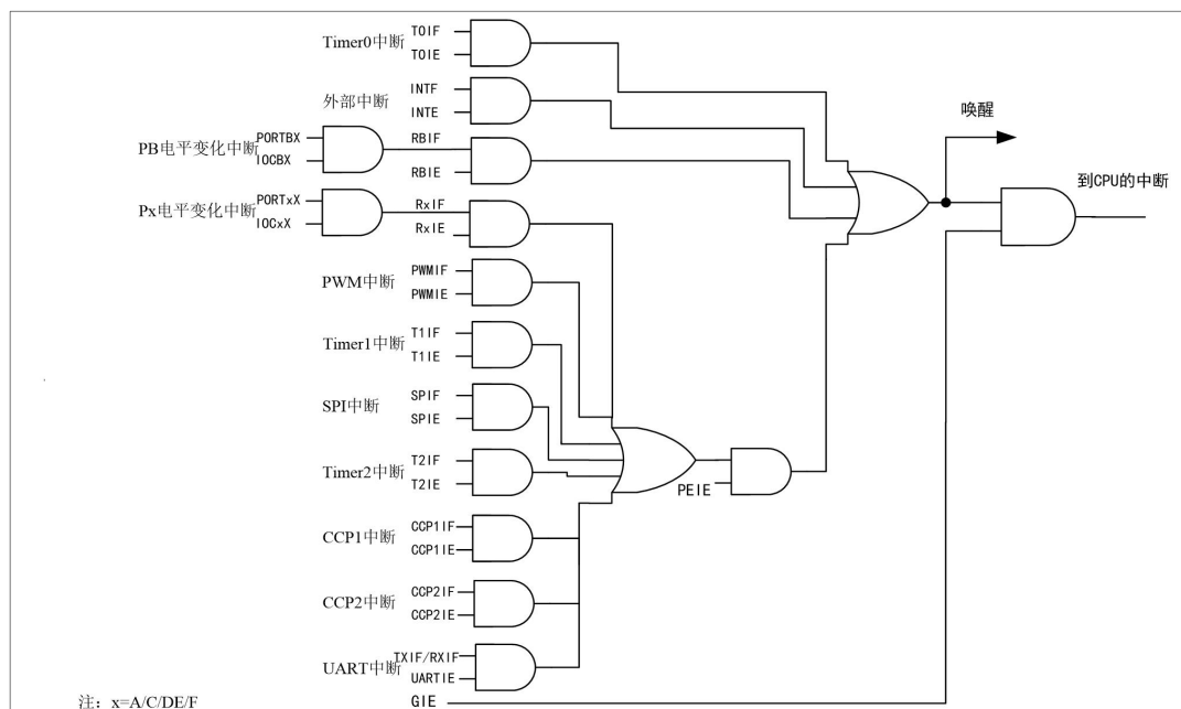
中断示意图
