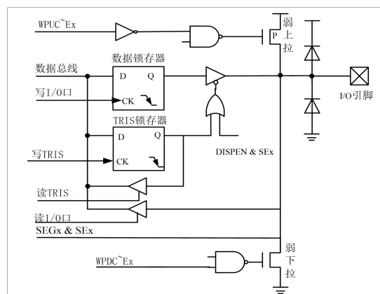
图 1- 6: PORTC、PORTD、PORTE 口等效电路
