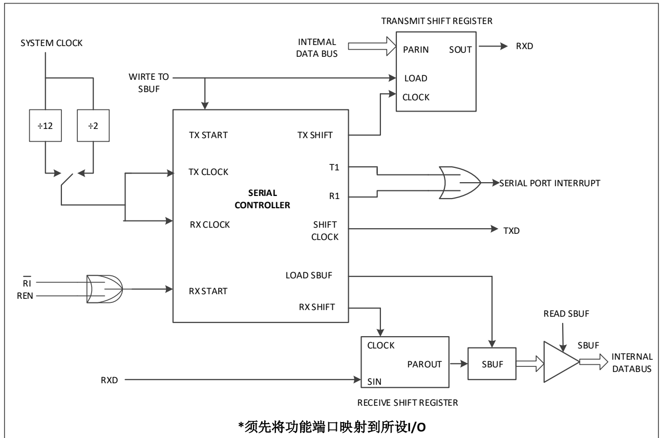
Figure 14-1 UART 模式 0 功能框图
