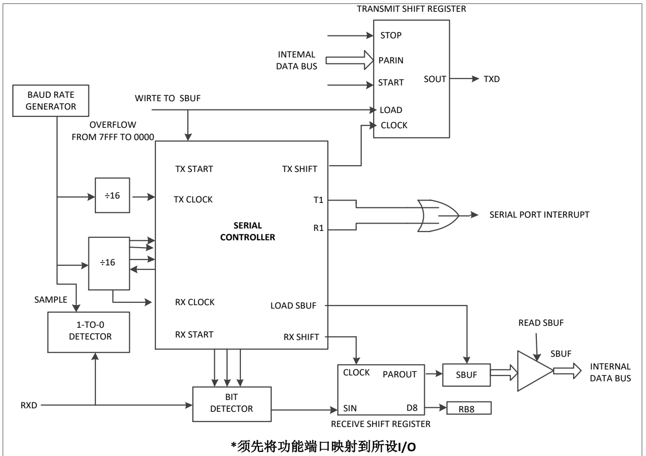
Figure 14-4 UART 模式 1 功能框图
