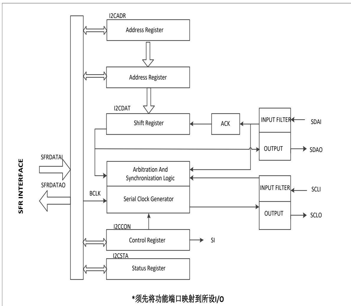
Figure 16-1 IIC 功能框图
