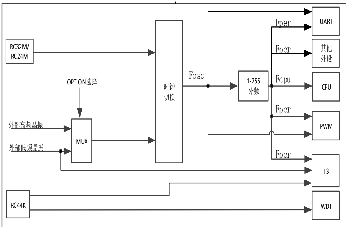
Figure 4-1 系统时钟框图
