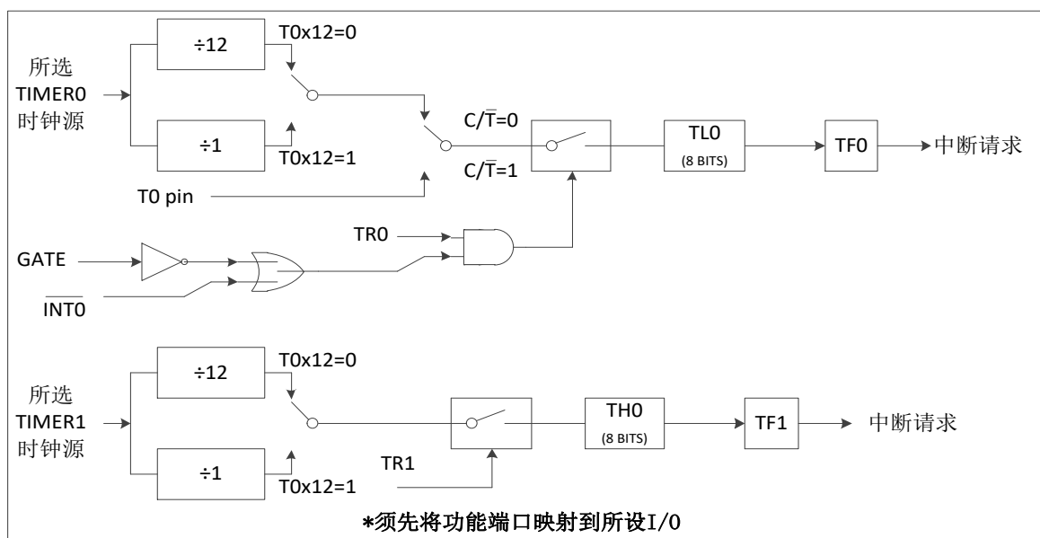
Figure 9-4 TIMER0 方式 3 功能框图
