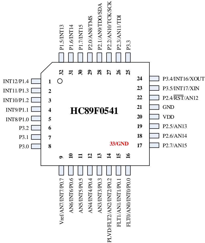
Figure 1-2 LQFP32/QFN32 引脚配置图 (QFN32 底衬与 PIN21(GND)相连)
