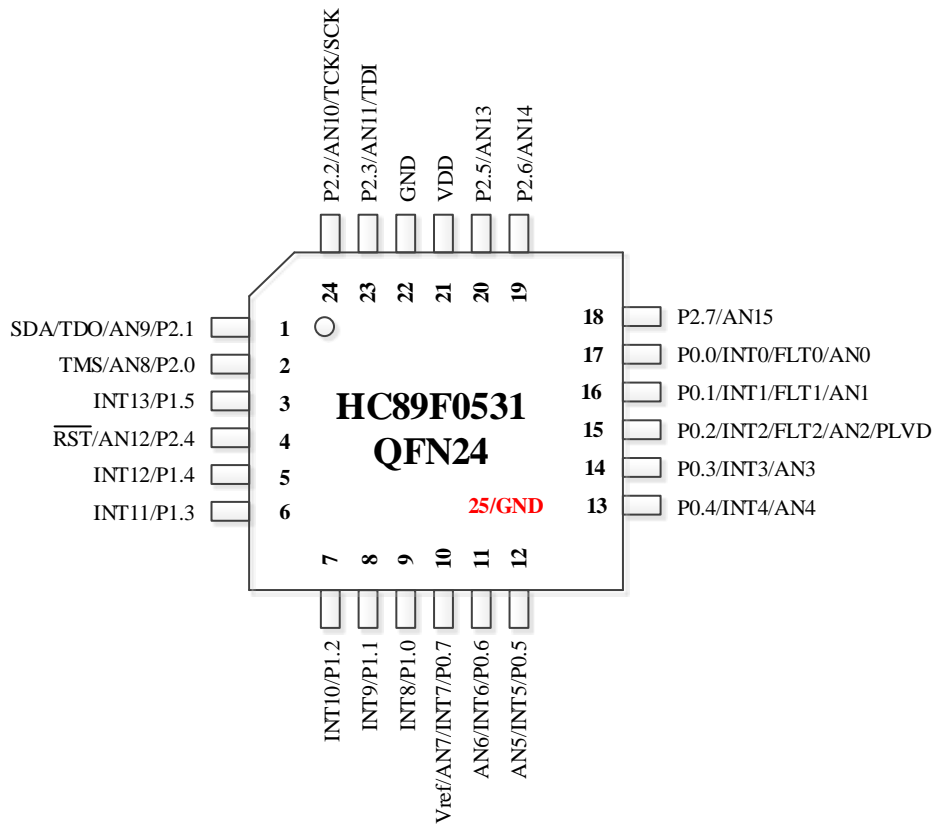
Figure 1-5 QFN24 引脚配置图 (底衬与 PIN22(GND)相连)
