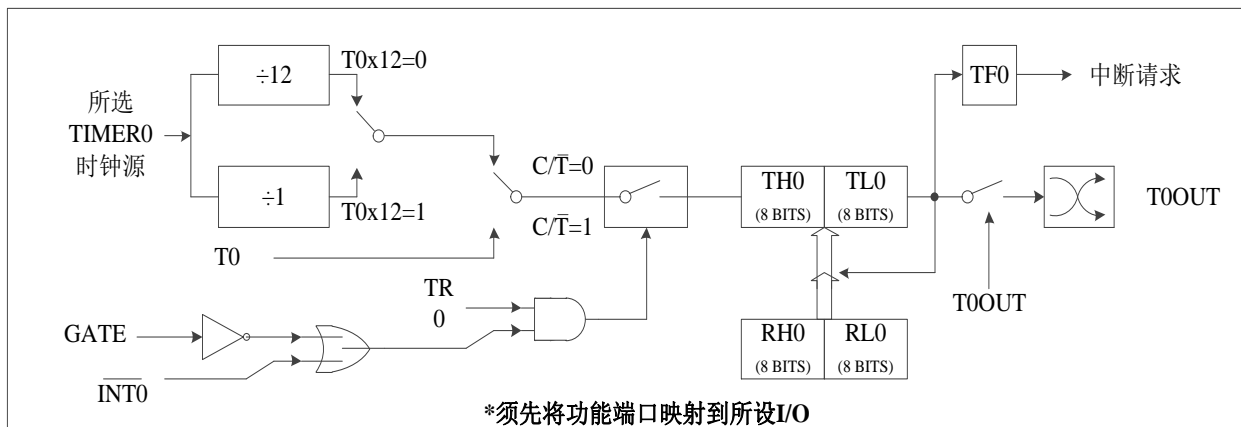
Figure 9-1 TIMER0 方式 0 功能框图
