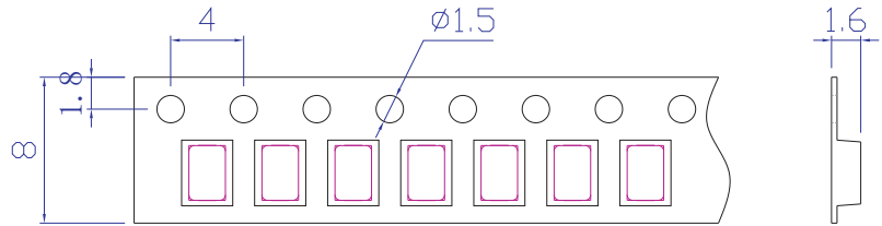
编带示意图
