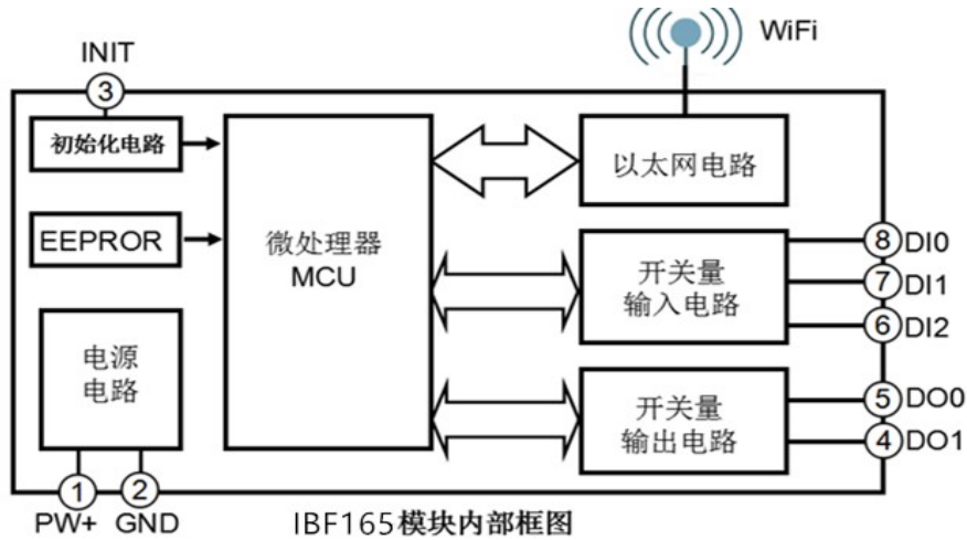
图 2 IBF165 模块内部框图
