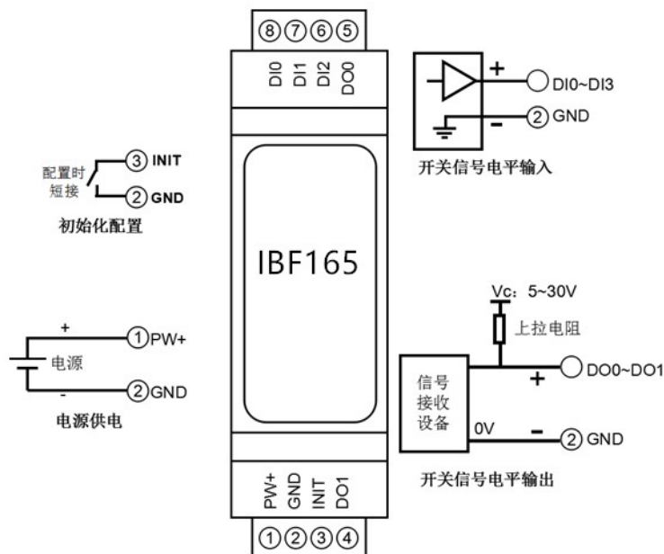
图 5 IBF165 模块接线图
