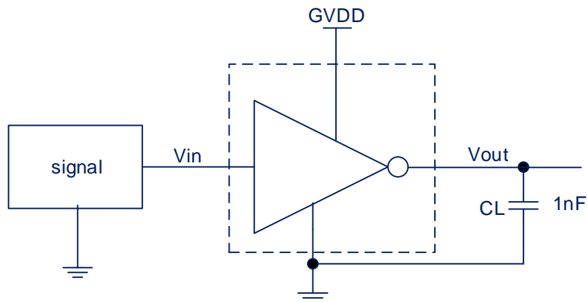
测试电路框图
