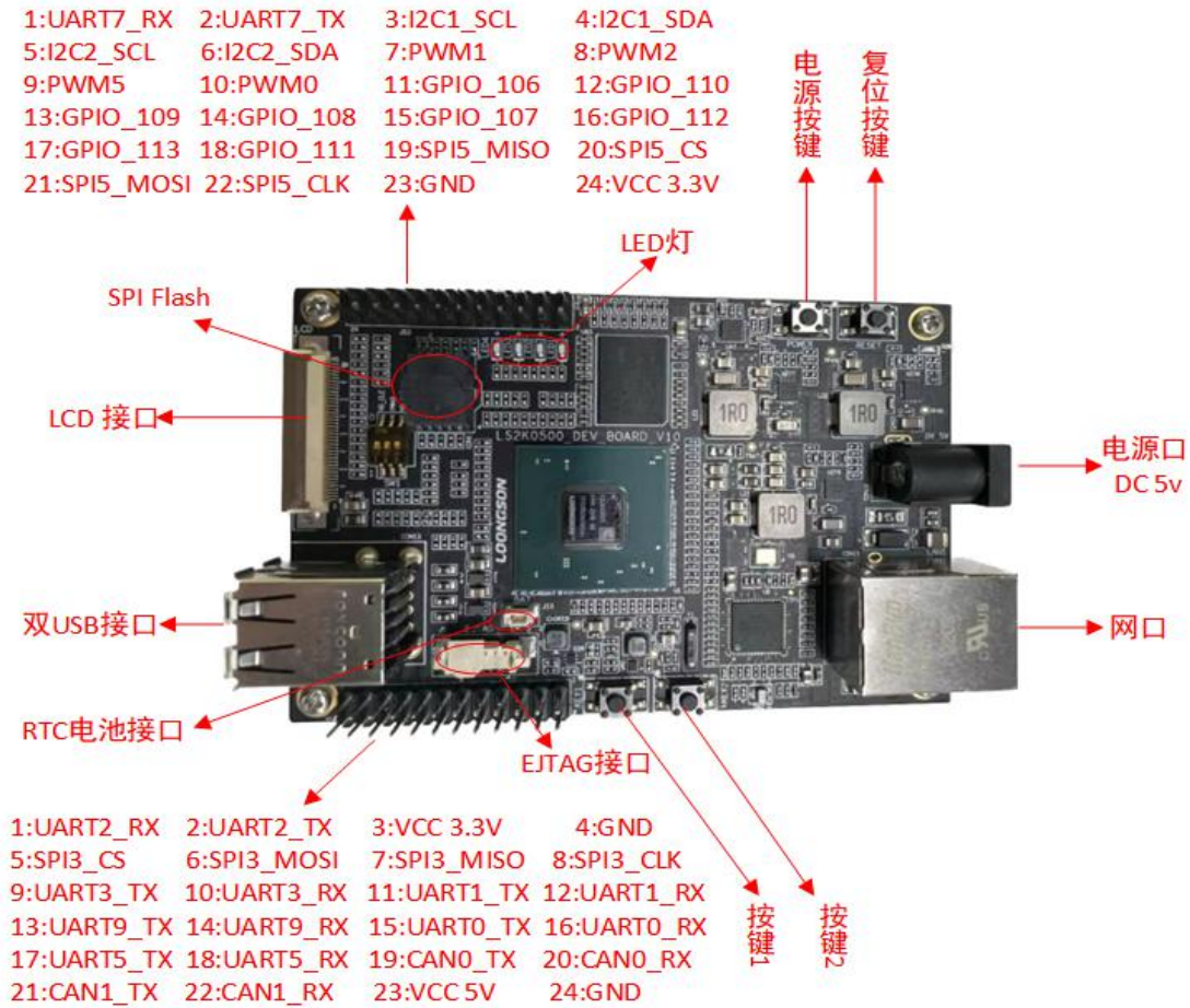
广东龙芯 2K500 先锋板接口图
