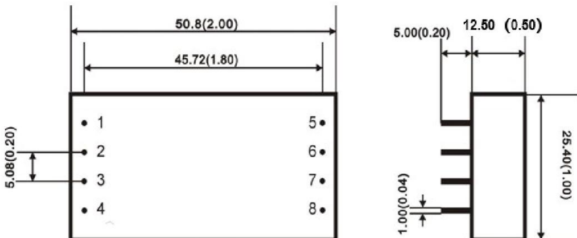
底视图侧视图 1
