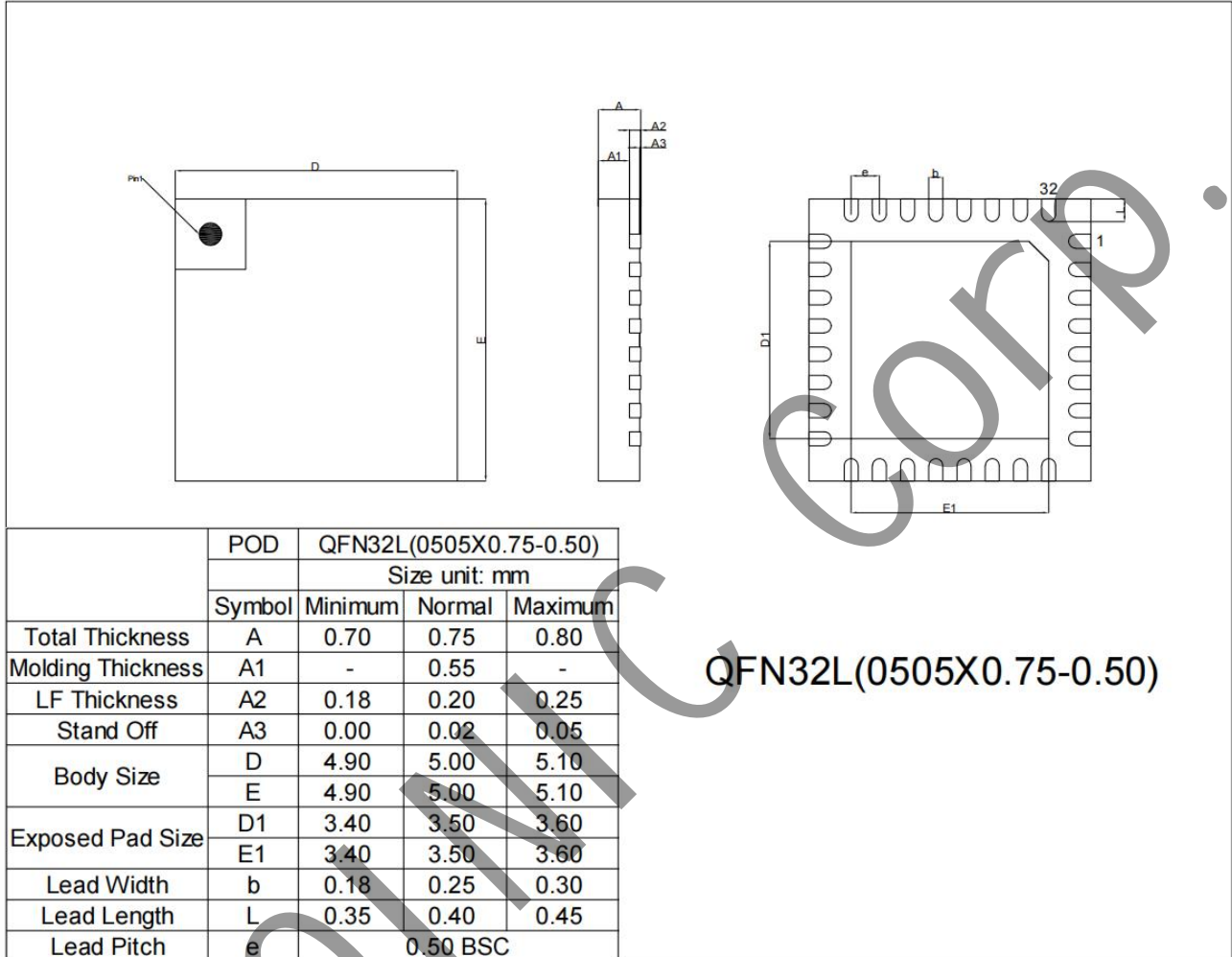
图 10 封装图
