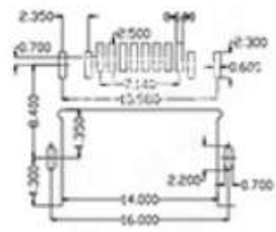
PCB参考图
