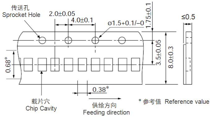
QN0603 系列 QN0603 series
