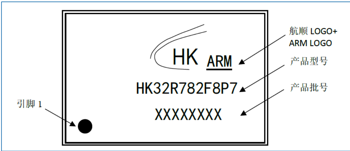
图 7-8 TSSOP20 丝印示例
