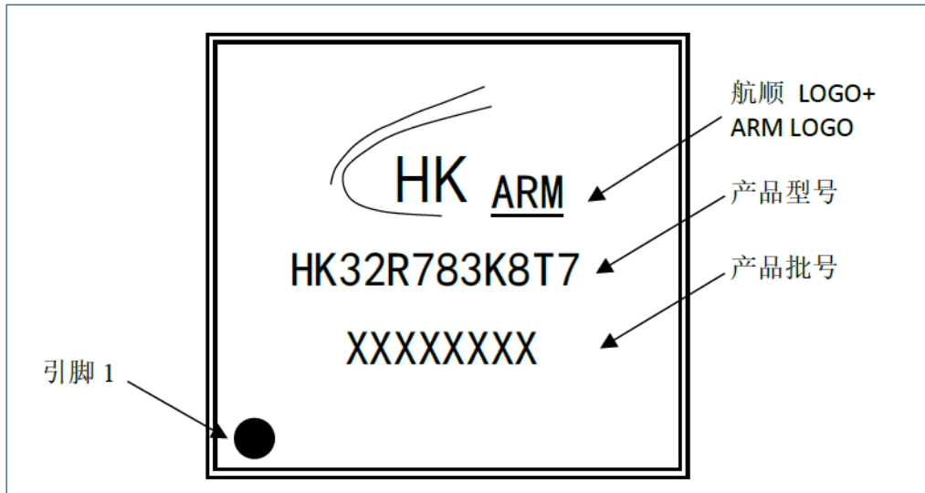
图 7-6 LQFP32 丝印示例
