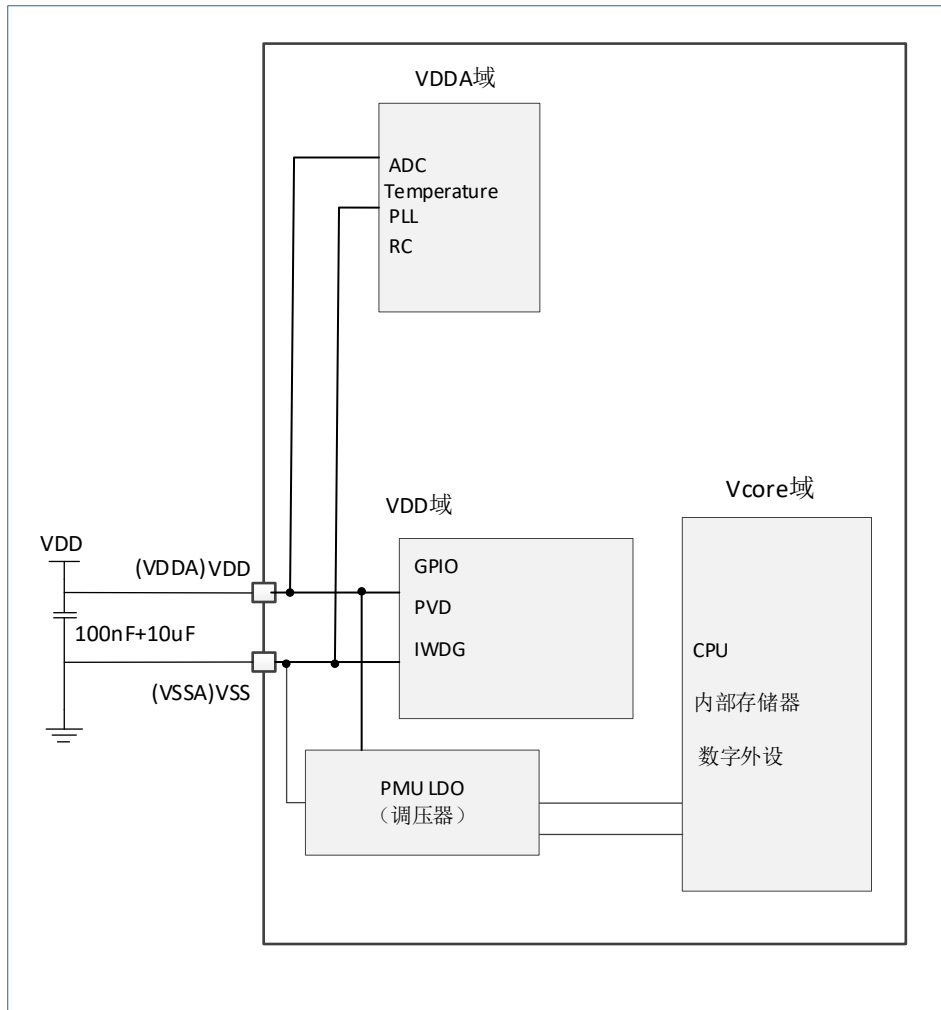
图 5-1 电源框图
