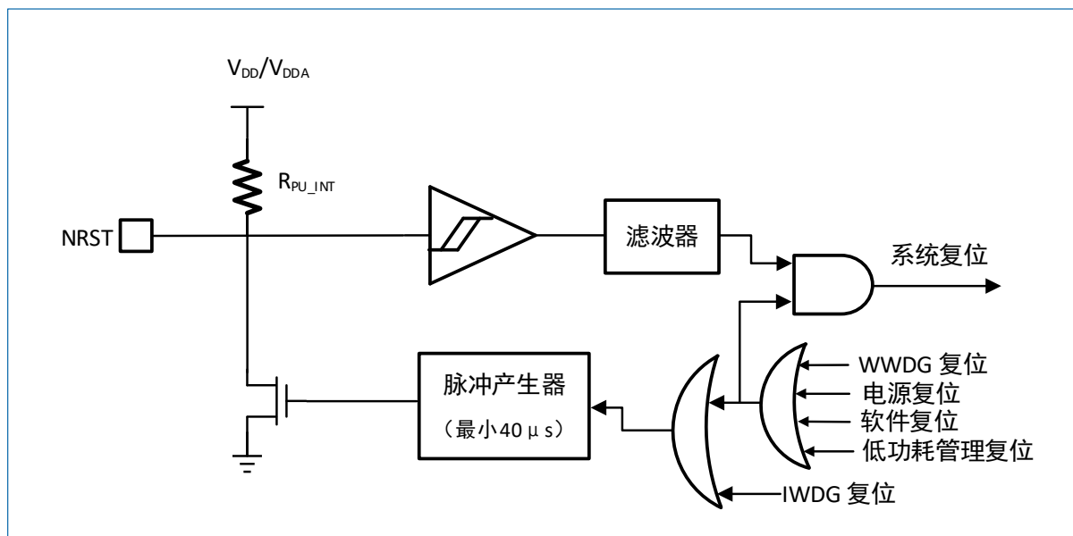
图 3-3 复位信号
