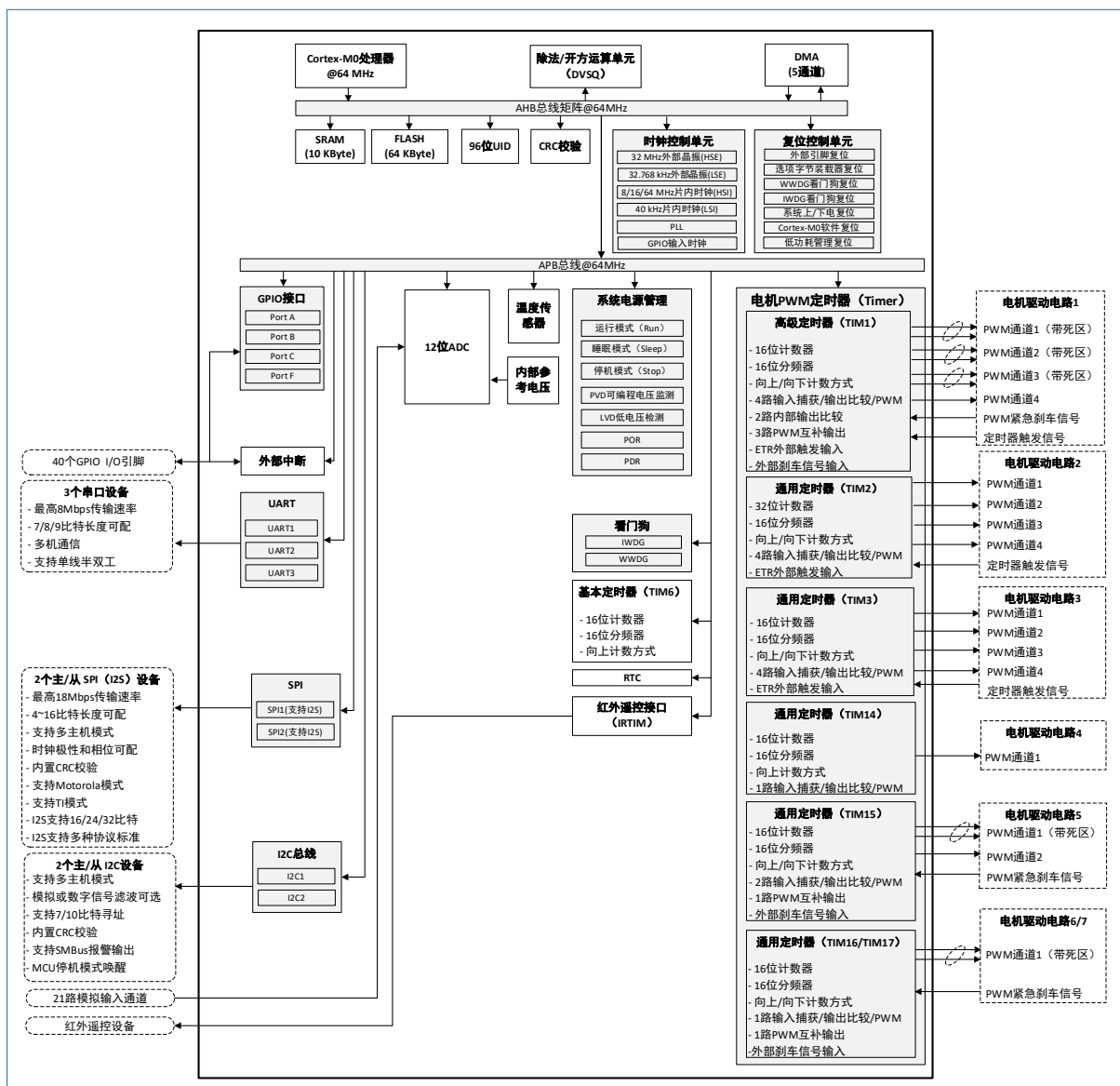
图 3-1 HK32R783S8T7 功能框图
