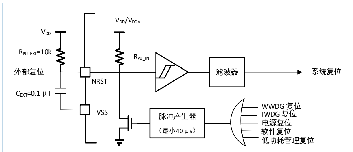
图 3-3 复位信号
