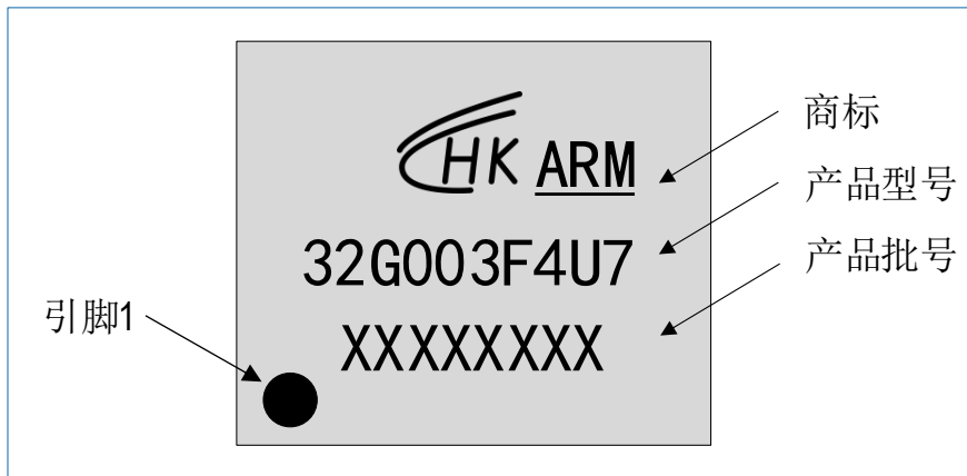
图 7-10 QFN20 HK32G003F4U7 丝印示例
