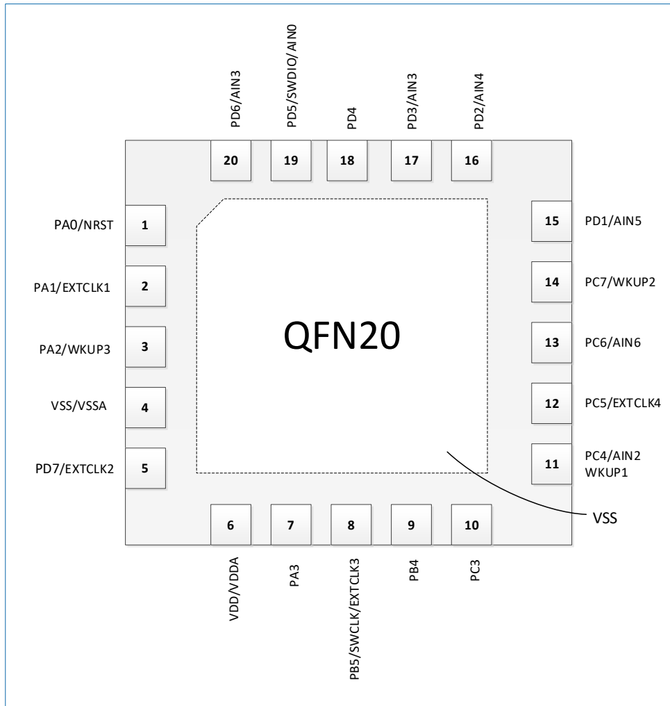
图 6-4 QFN20 封装管脚排列
