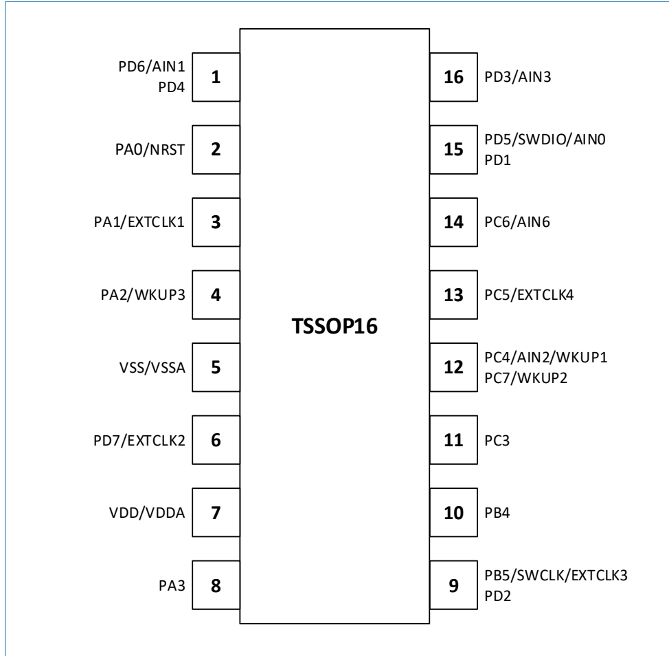
图 6-2 TSSOP16 封装管脚排列
