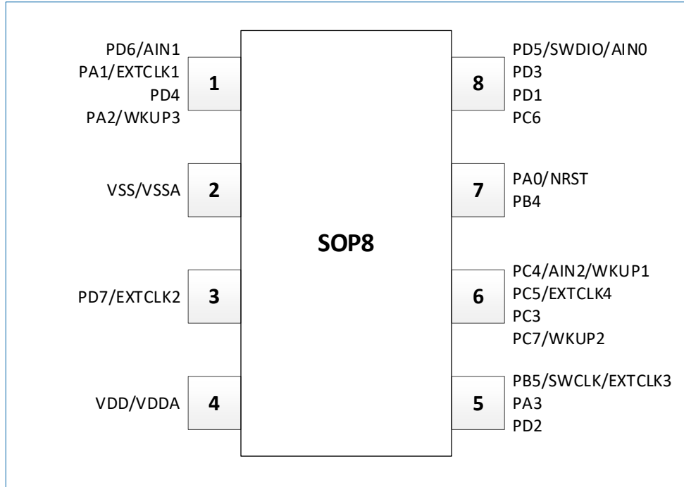
图 6-1 SOP8 封装管脚排列
