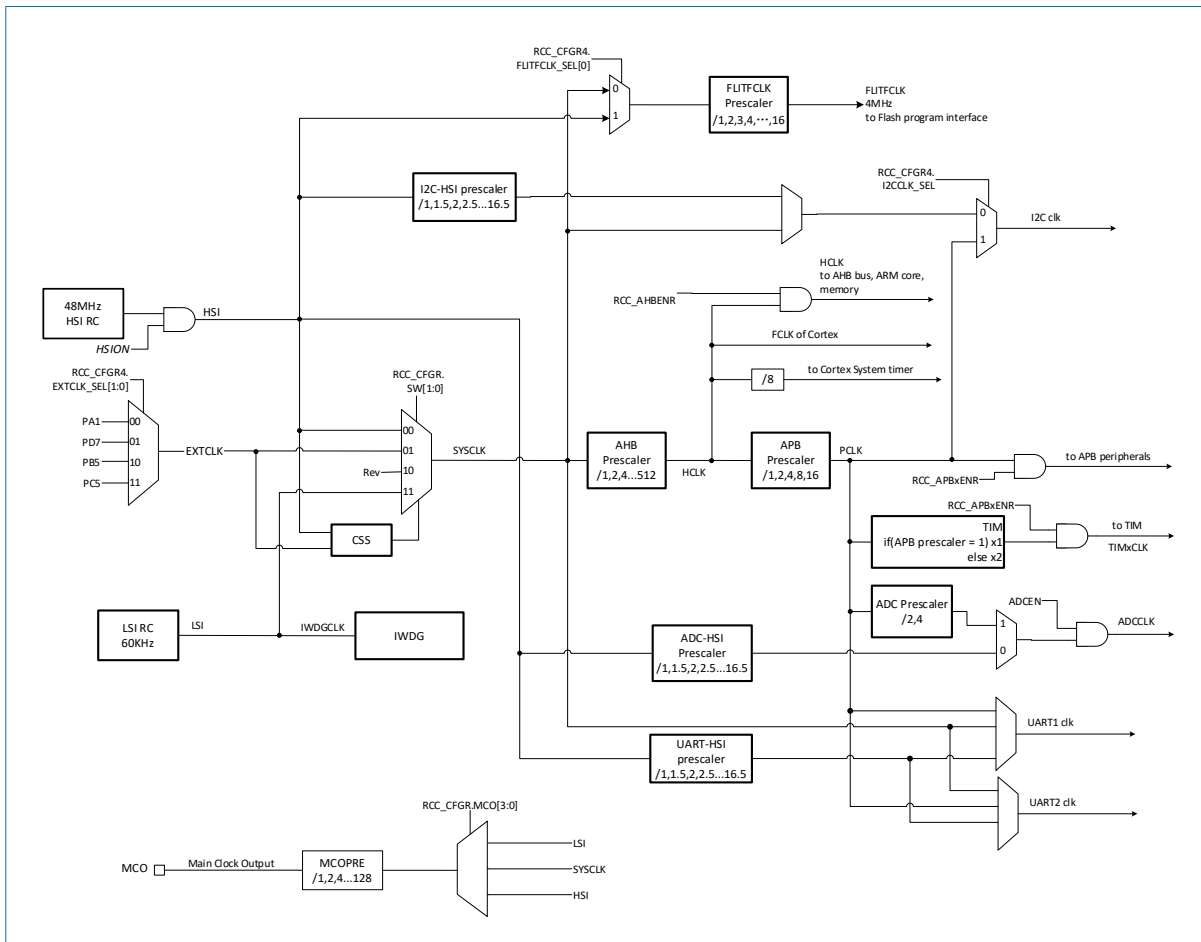
图 3-4 HK32G003 时钟树
