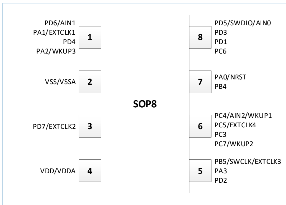
图 3-5 SOP8 封装的管脚排列
