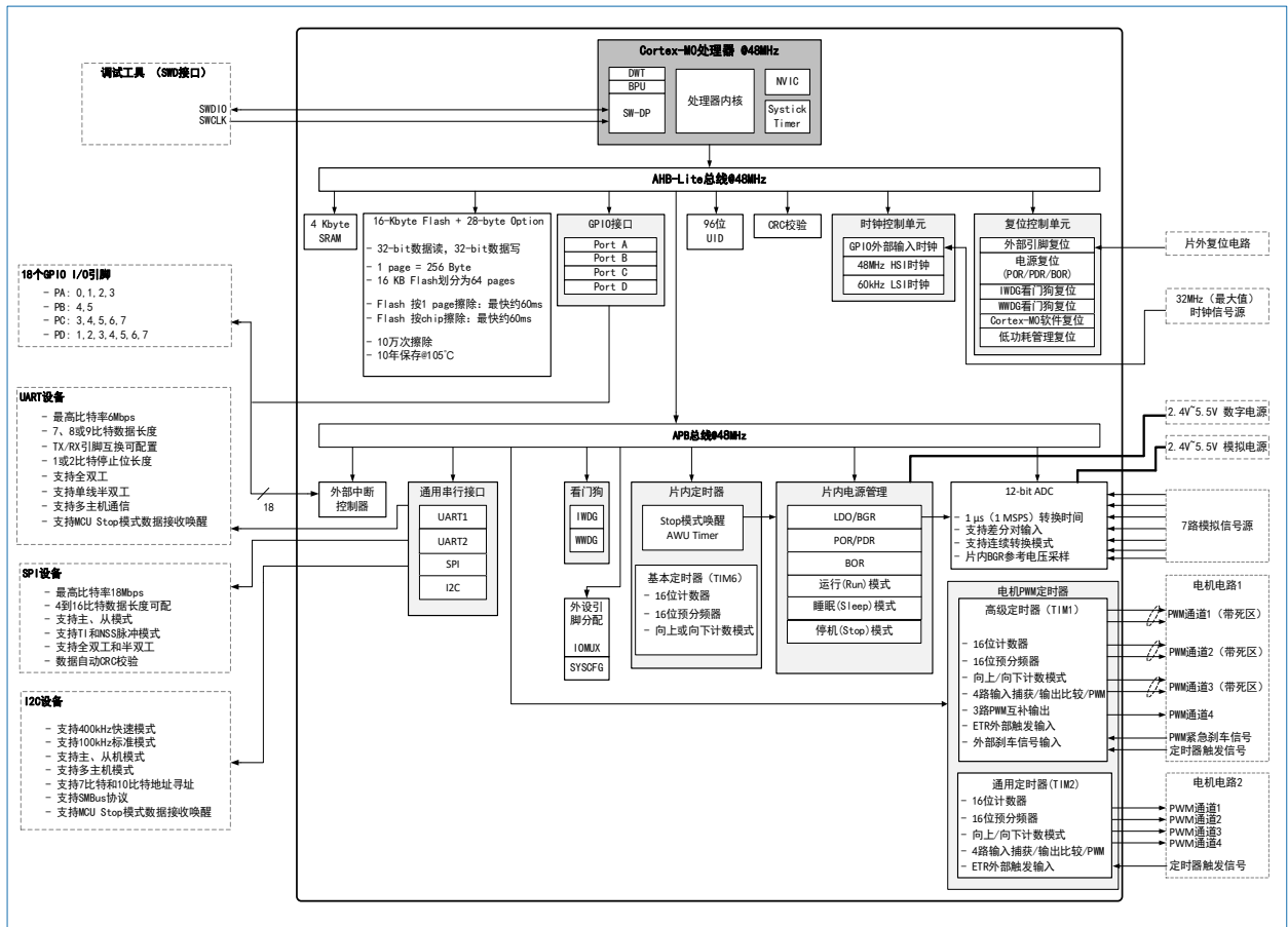
图 3-1 HK32G003 系统架构图
