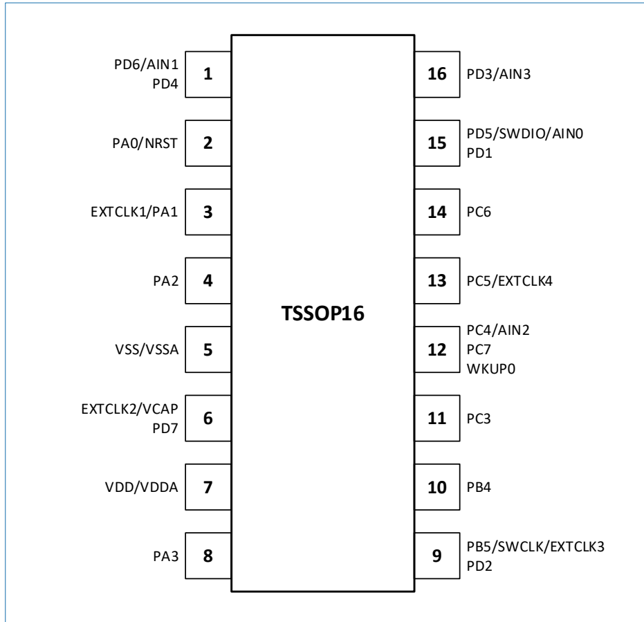
图 6-3 TSSOP16 封装
