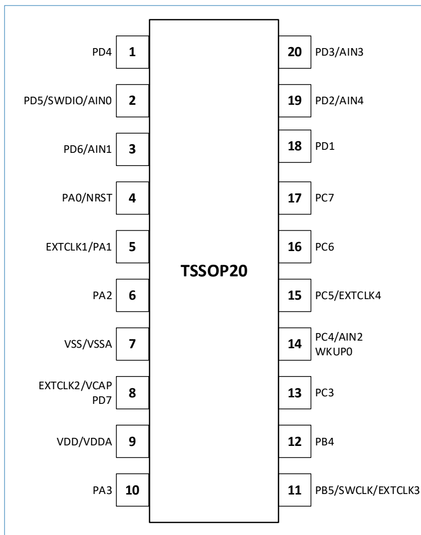
图 6-2 TSSOP20 封装
