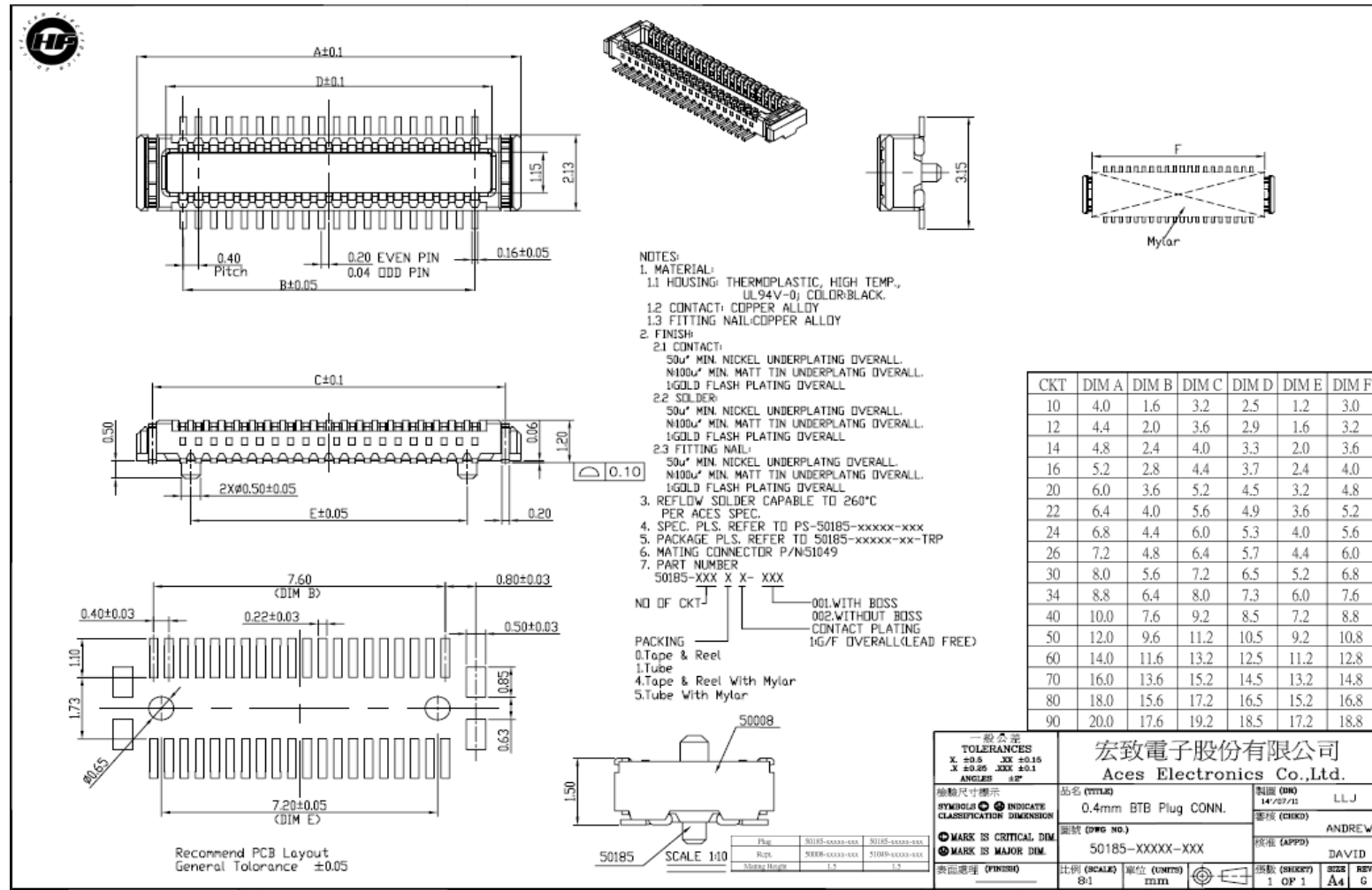
图 25 模块上使用的 BTB 连接器尺寸信息
