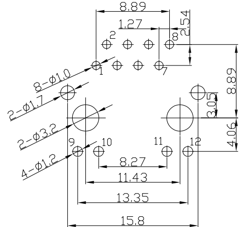
P.C.B参考图
