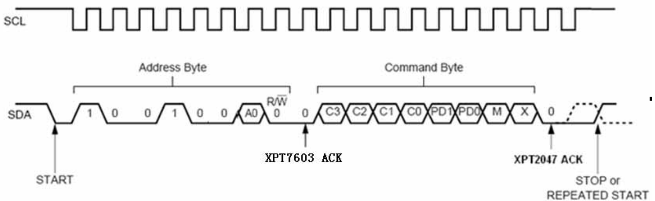
图 12 I2C 接口写命令时序图
