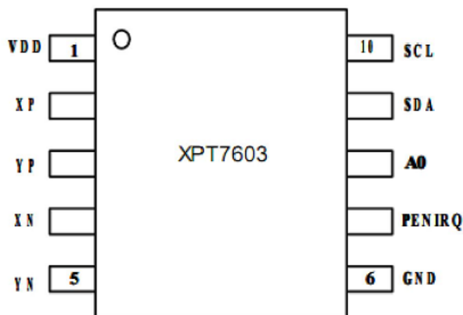
XPT7603 MSOP-10 封装的管脚分布图
