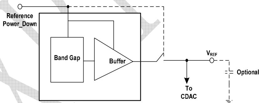
图 6 内部电压源示意图
