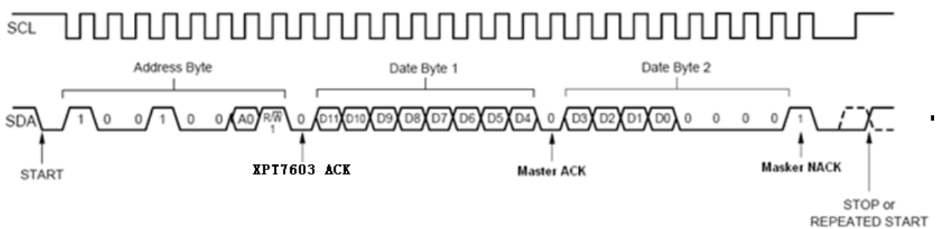
图 13 I2C 接口读命令时序图
