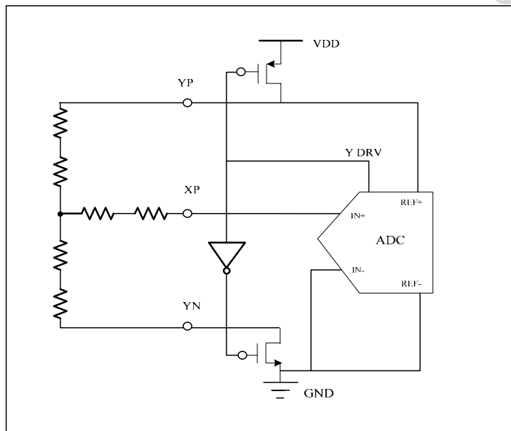
图 8 差分参考源工作模式简图 (C3=1, Y 方向驱动开关闭合, XP 作为模拟输入)
