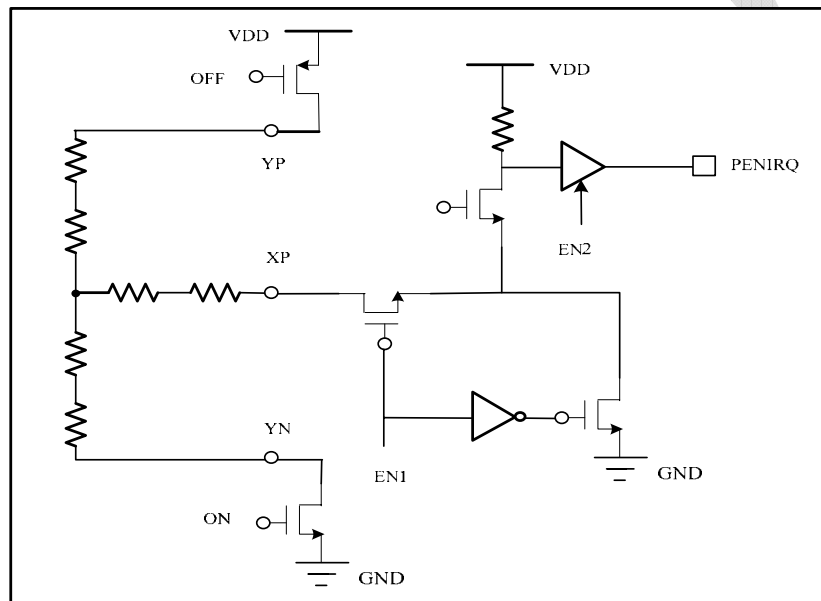
图 16 PENIRQ 功能模块图
