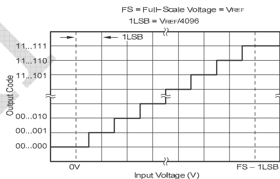
图 15 理想情况输入电压和输出编码对应关系
