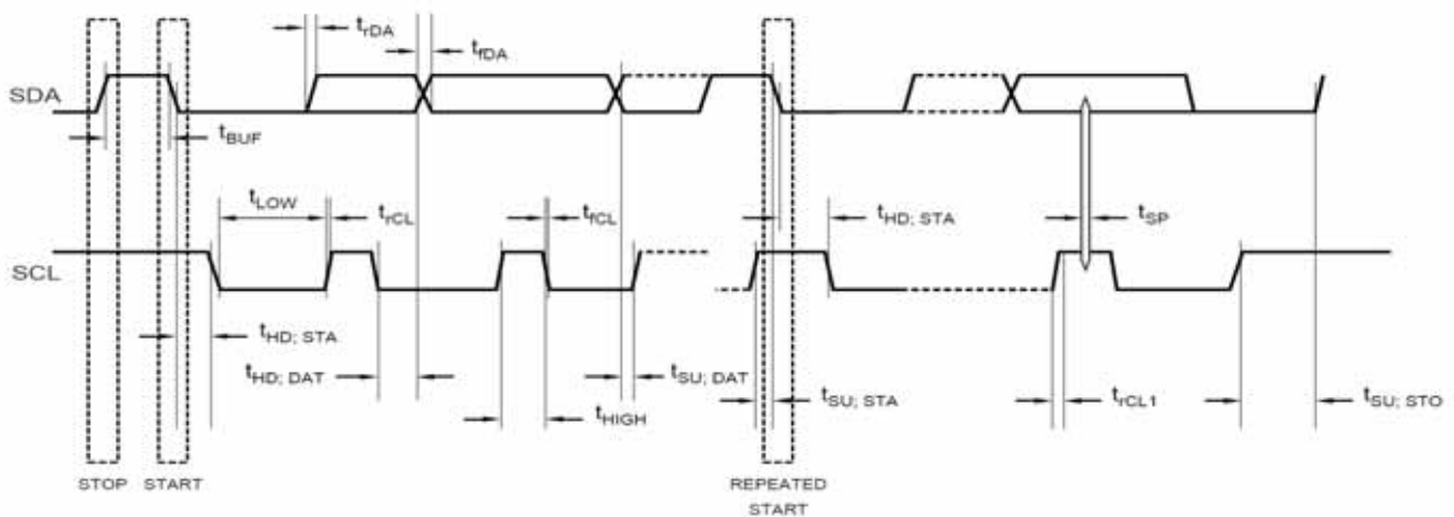
图 14 XPT7603 数字接口时序图
