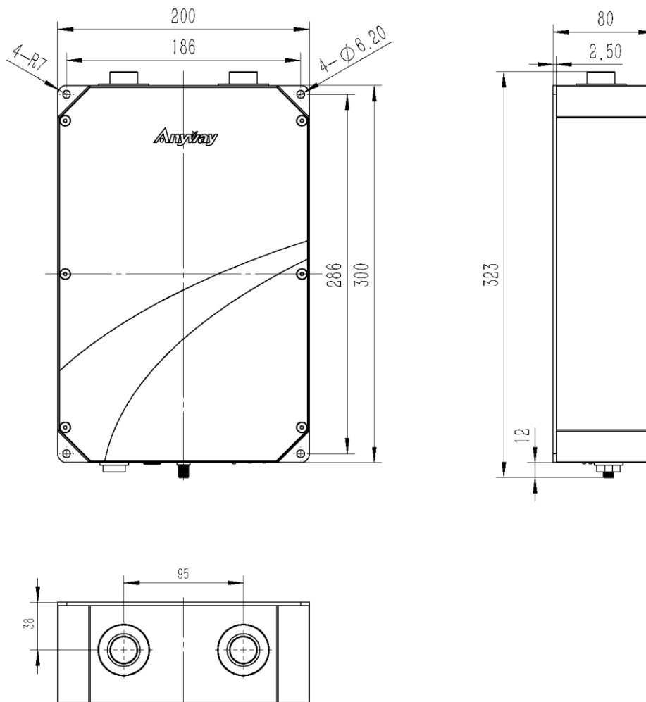
图 1 外形图
