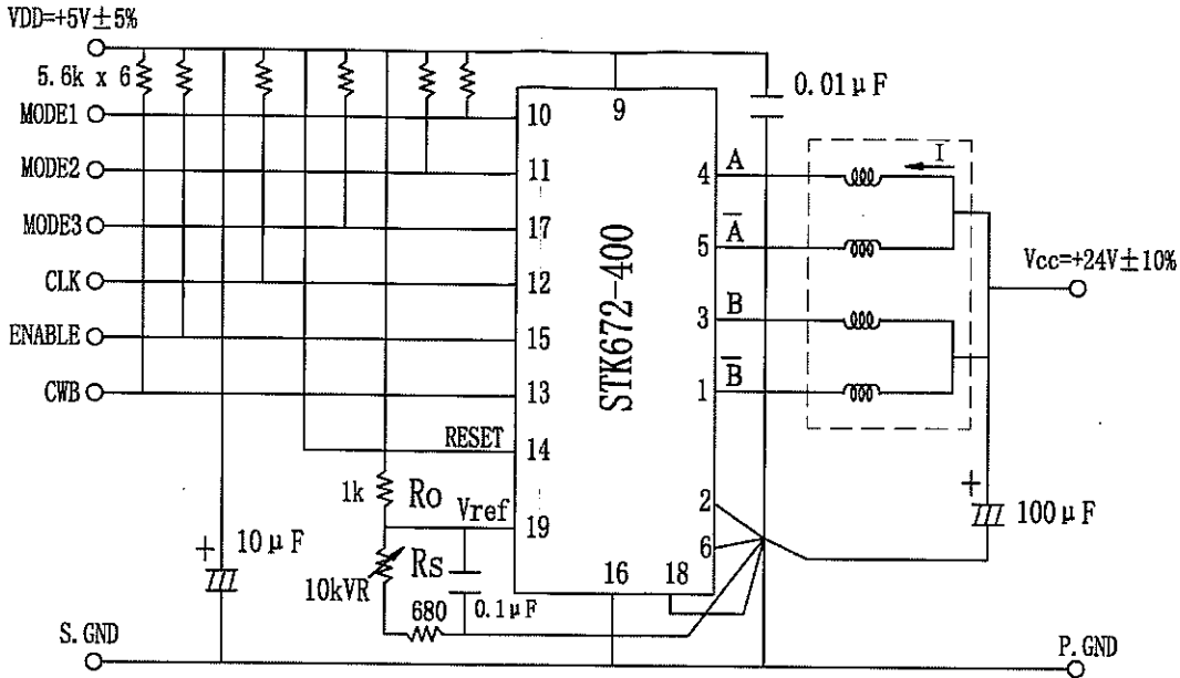
图1 实验电路 FIG1. TEST CIRCUIT
