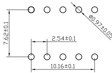
PCB开孔
