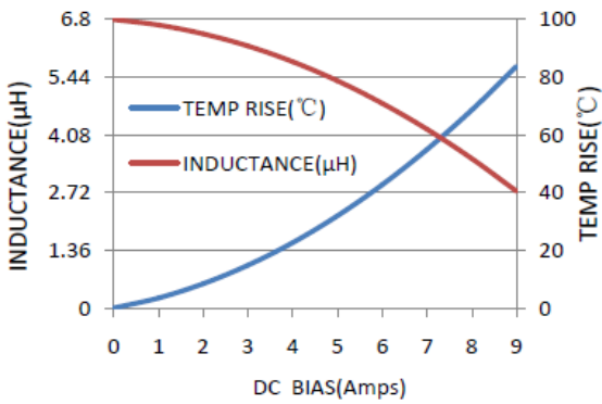
FSA0630-100MT
