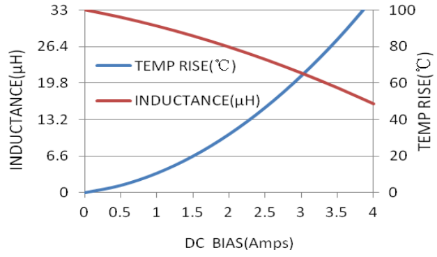
FSA0630-330MT
