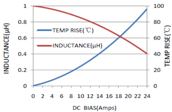
FSA0630-1R0MT
