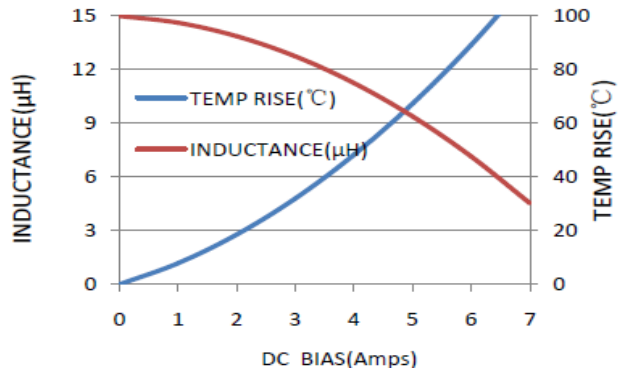
FSA0630-150MT
