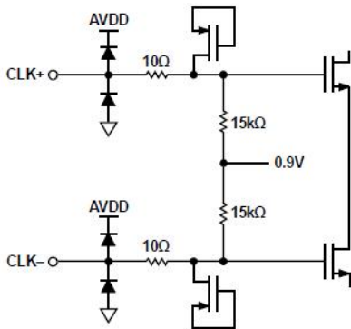
图 9. 等效时钟输入电路
