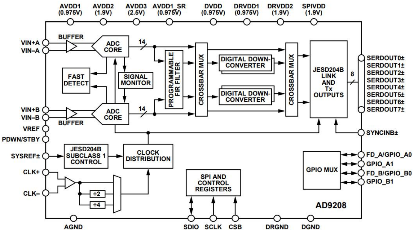
图 2. 功能框图
