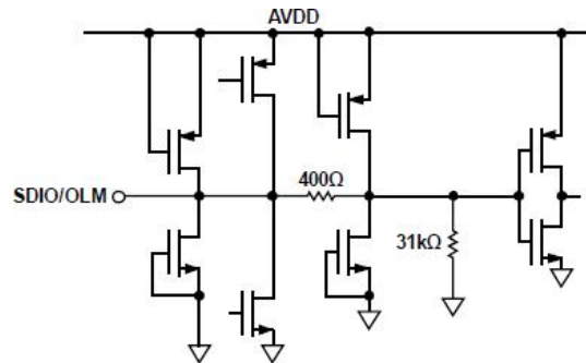
图 10. 等效 SDIO/OLM 输入电路
