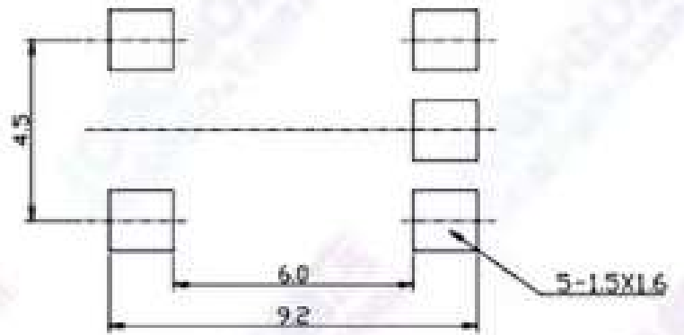
P.C.B LAYOUT
