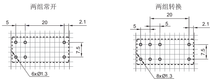
安装孔尺寸 (底视图)
