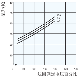
线圈温升
